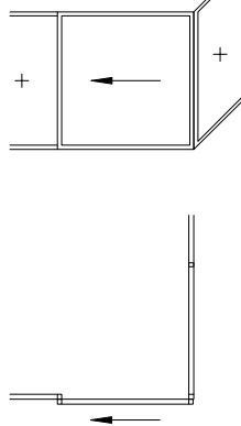
Angle externe avec montant
