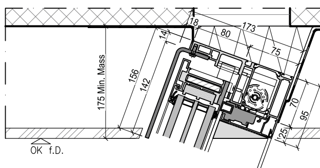
Schnitt B-B
