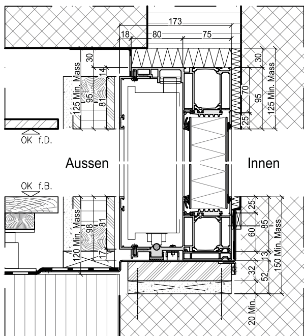
Schnitt B-B
