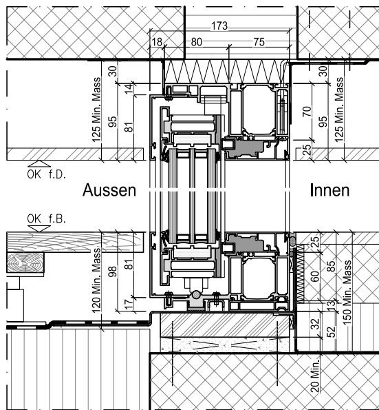
Schnitt B-B
