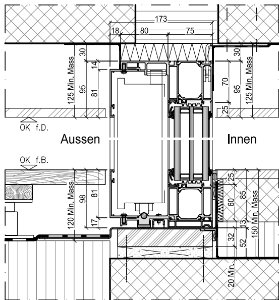
Schnitt A-A
