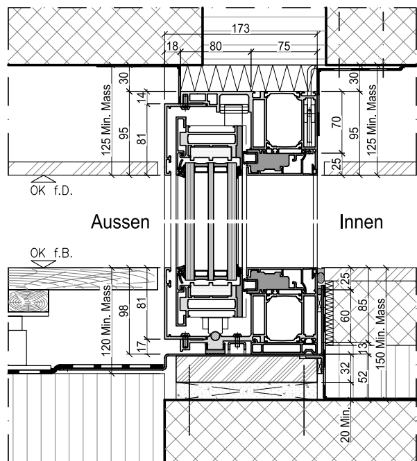
Schnitt B-B
