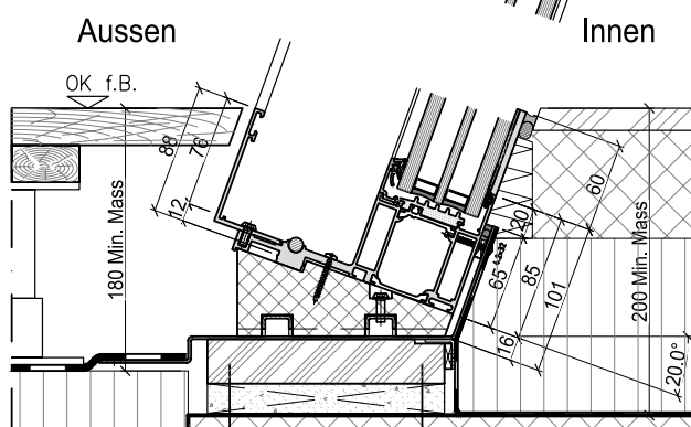
Schnitt C-C
