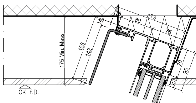
Schnitt A-A
