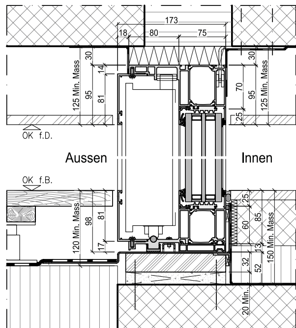
Schnitt A-A
