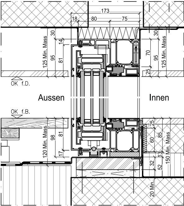
Schnitt B-B
