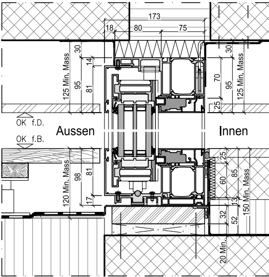
Schnitt C-C
