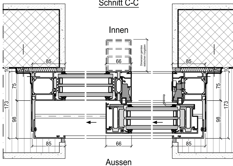
Schnitt C-C
