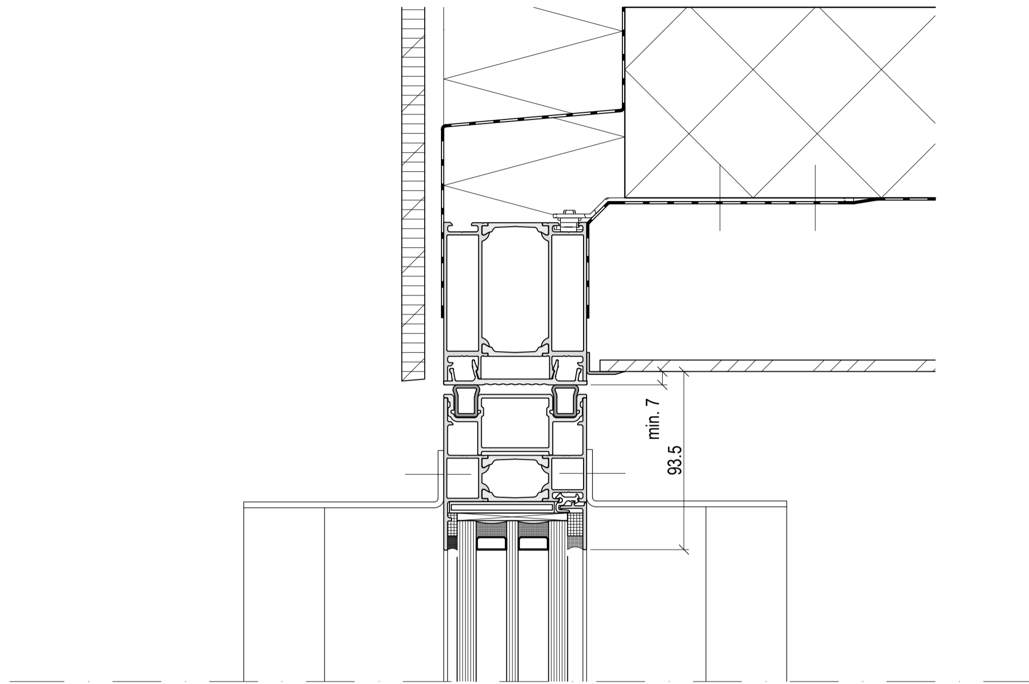
Detail A Maßstab = 1 : 2
