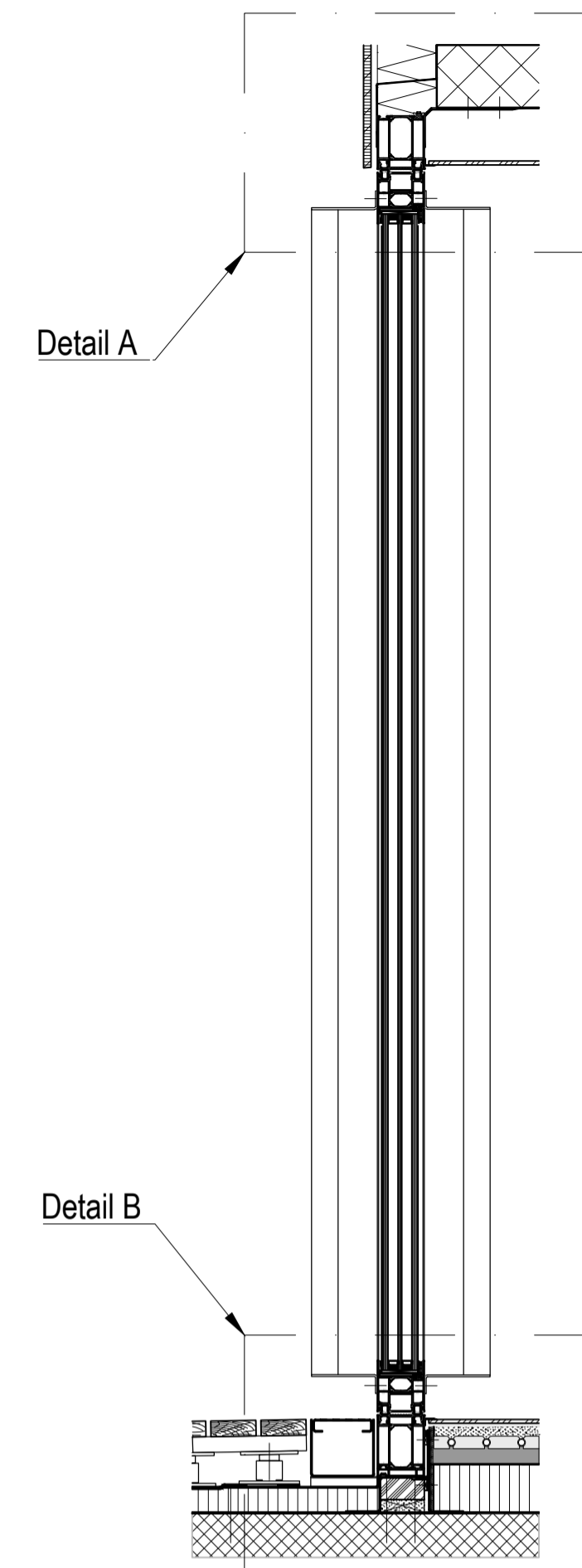
Schnitt A-A Maßstab = 1 : 10
