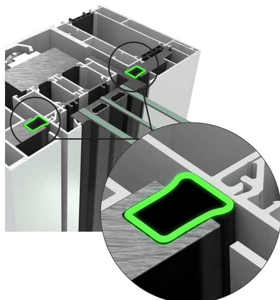
Airtight seal
