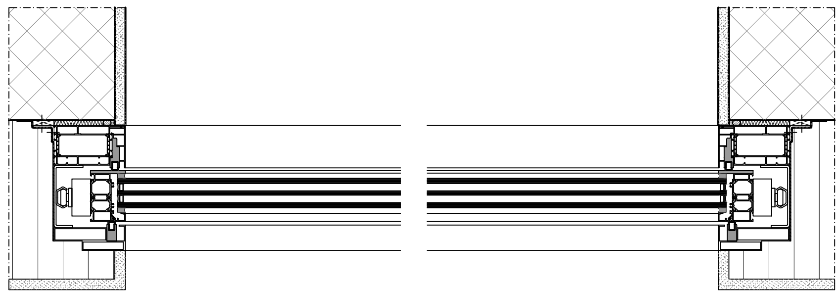
Schnitt B-B
