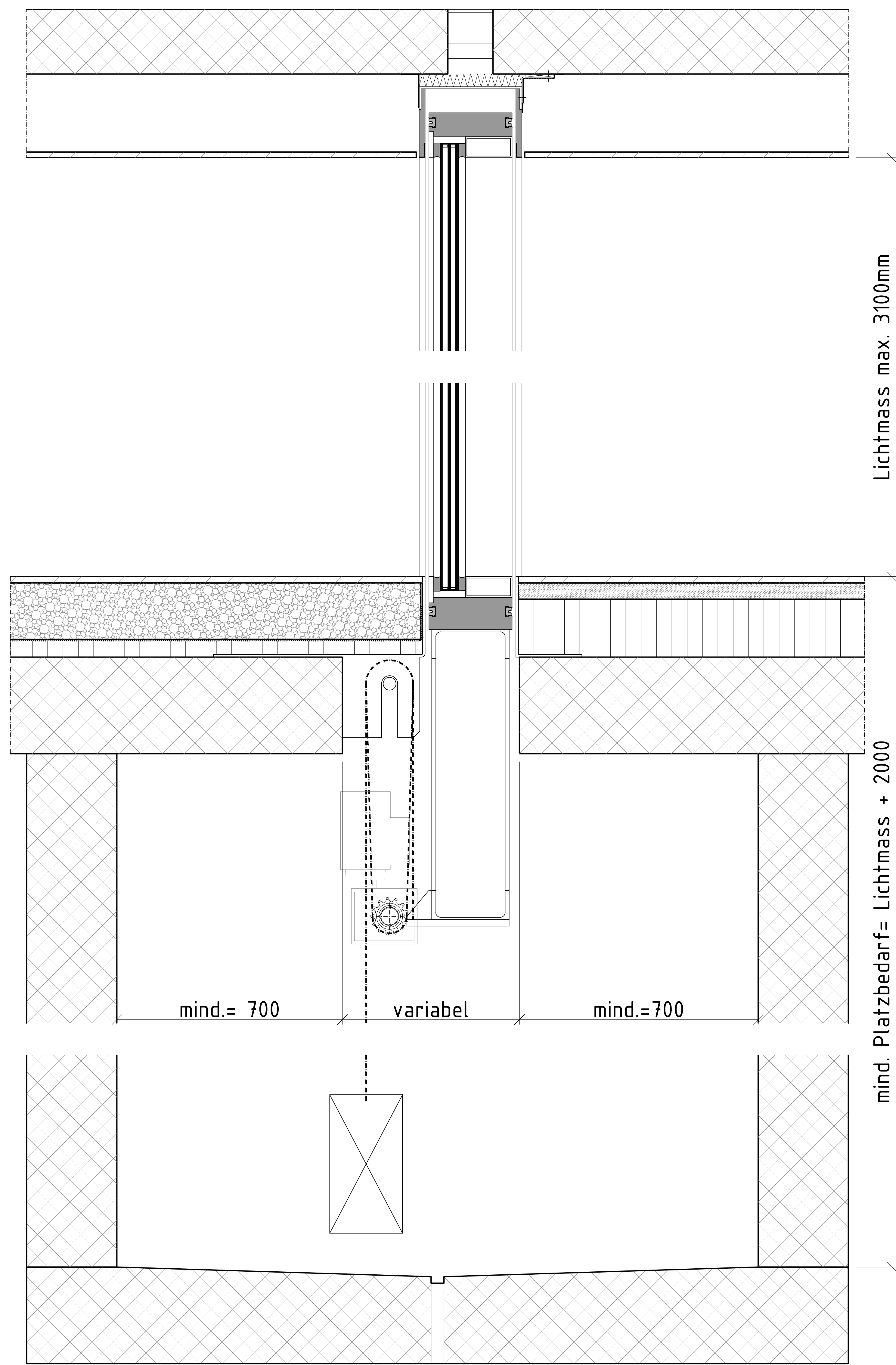
Schnitt A-A
