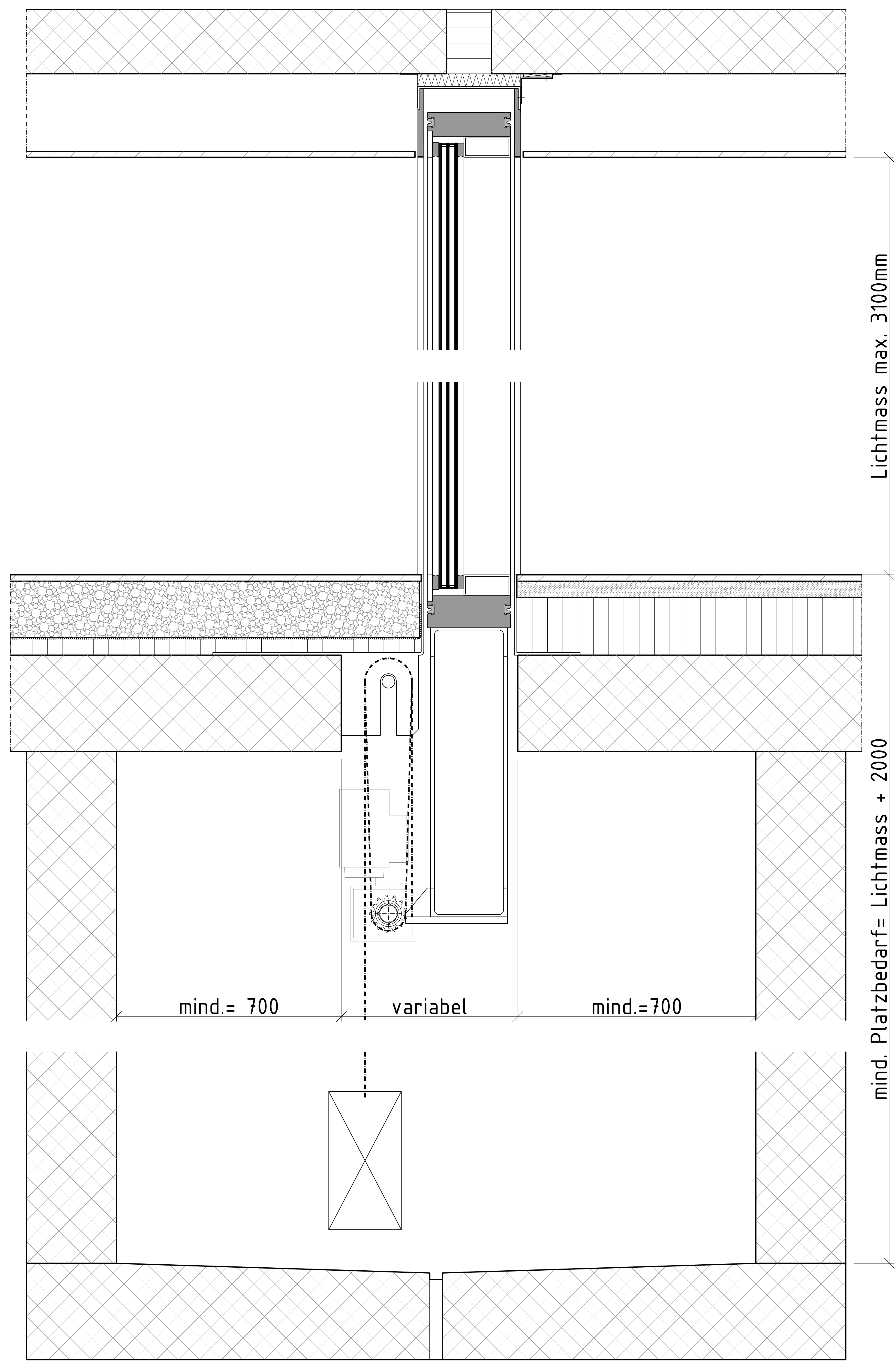
Schnitt A-A
