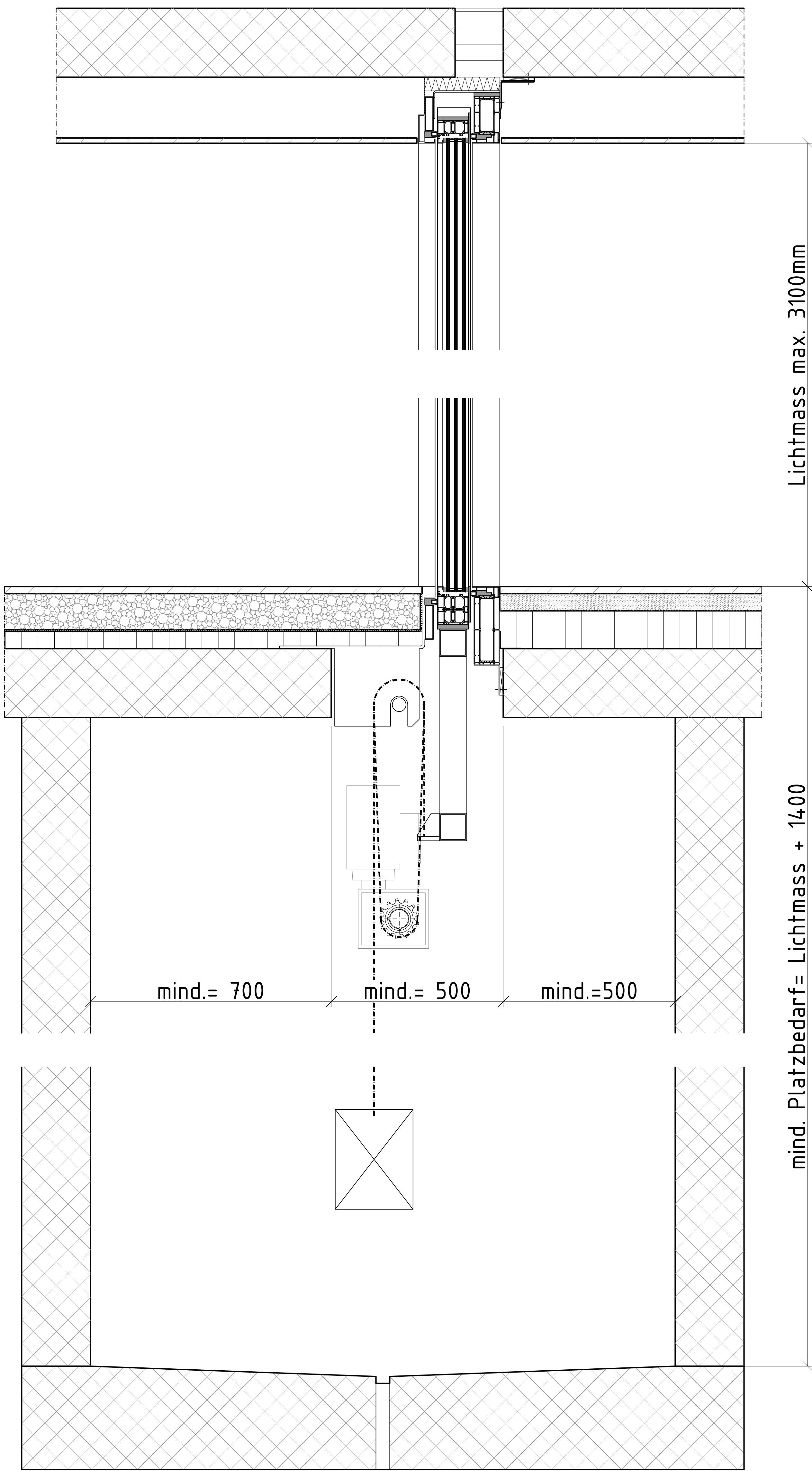
Schnitt A-A
