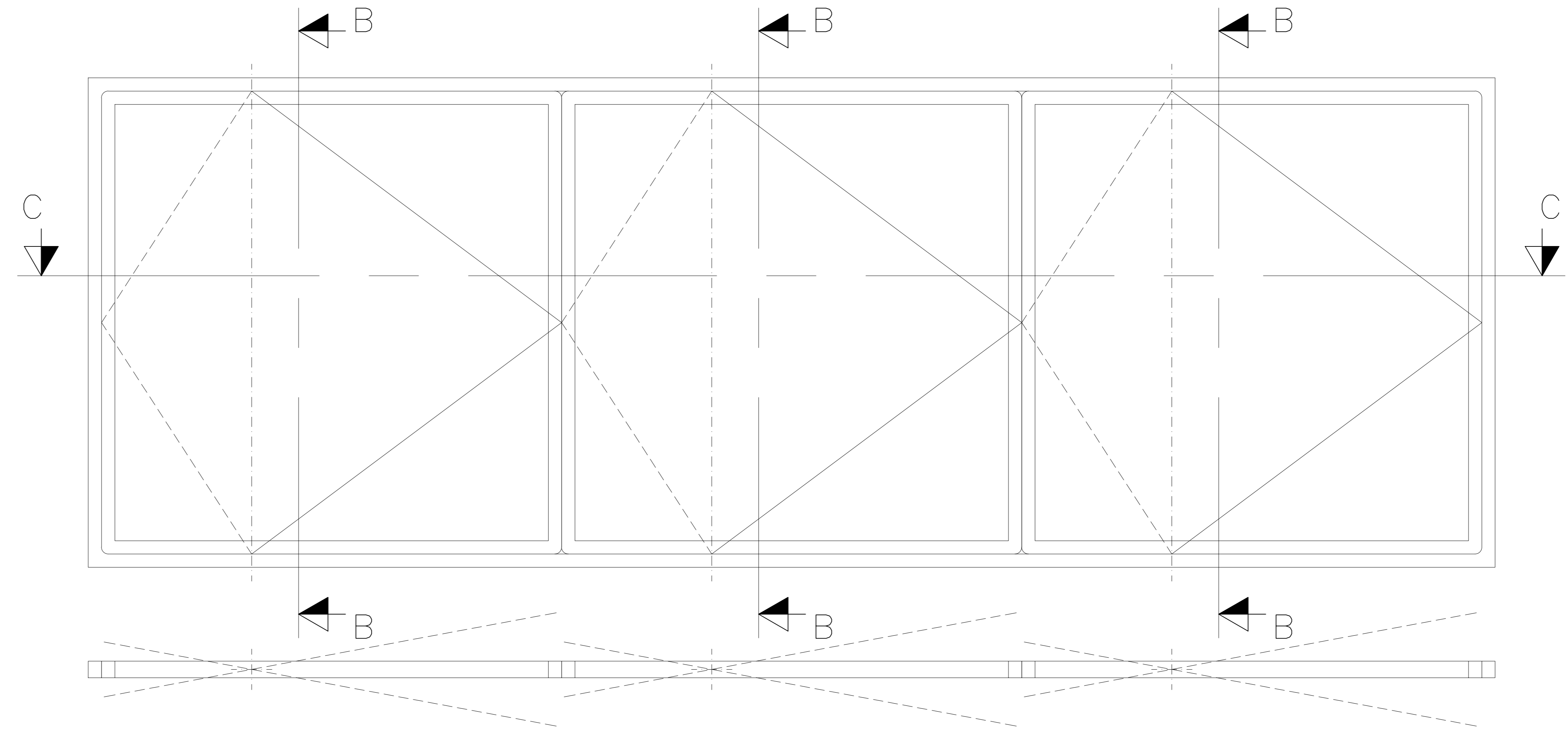
Ansicht
