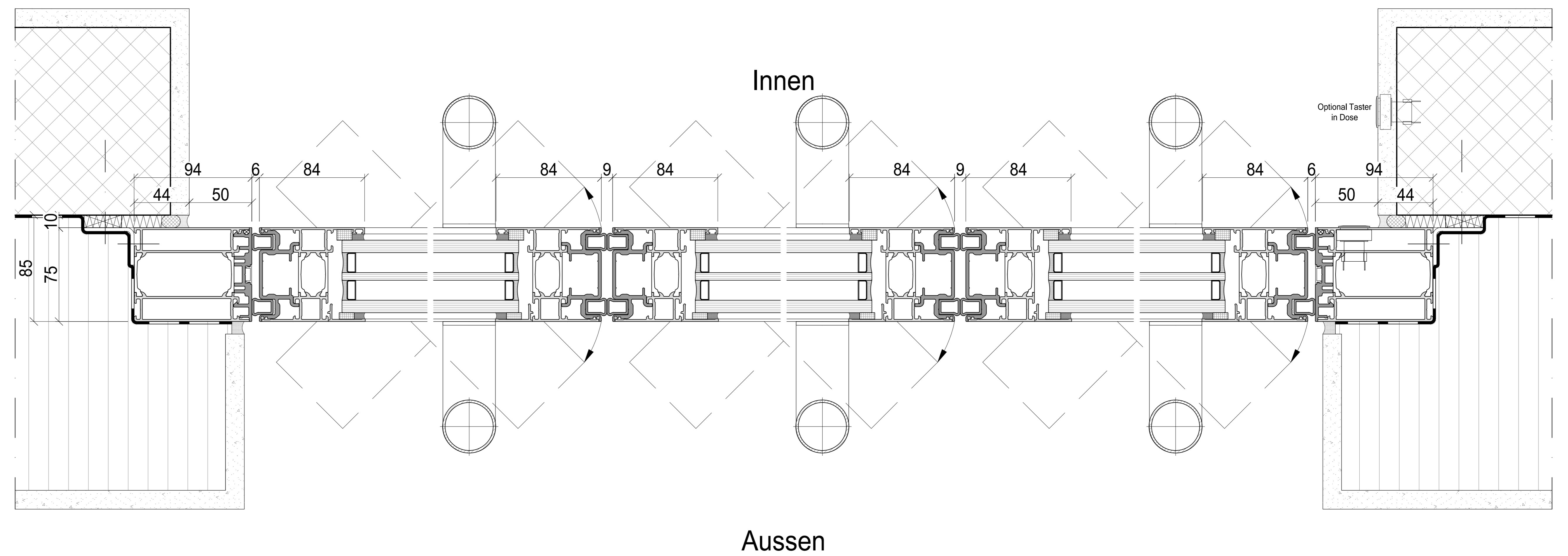
Schnitt C-C
