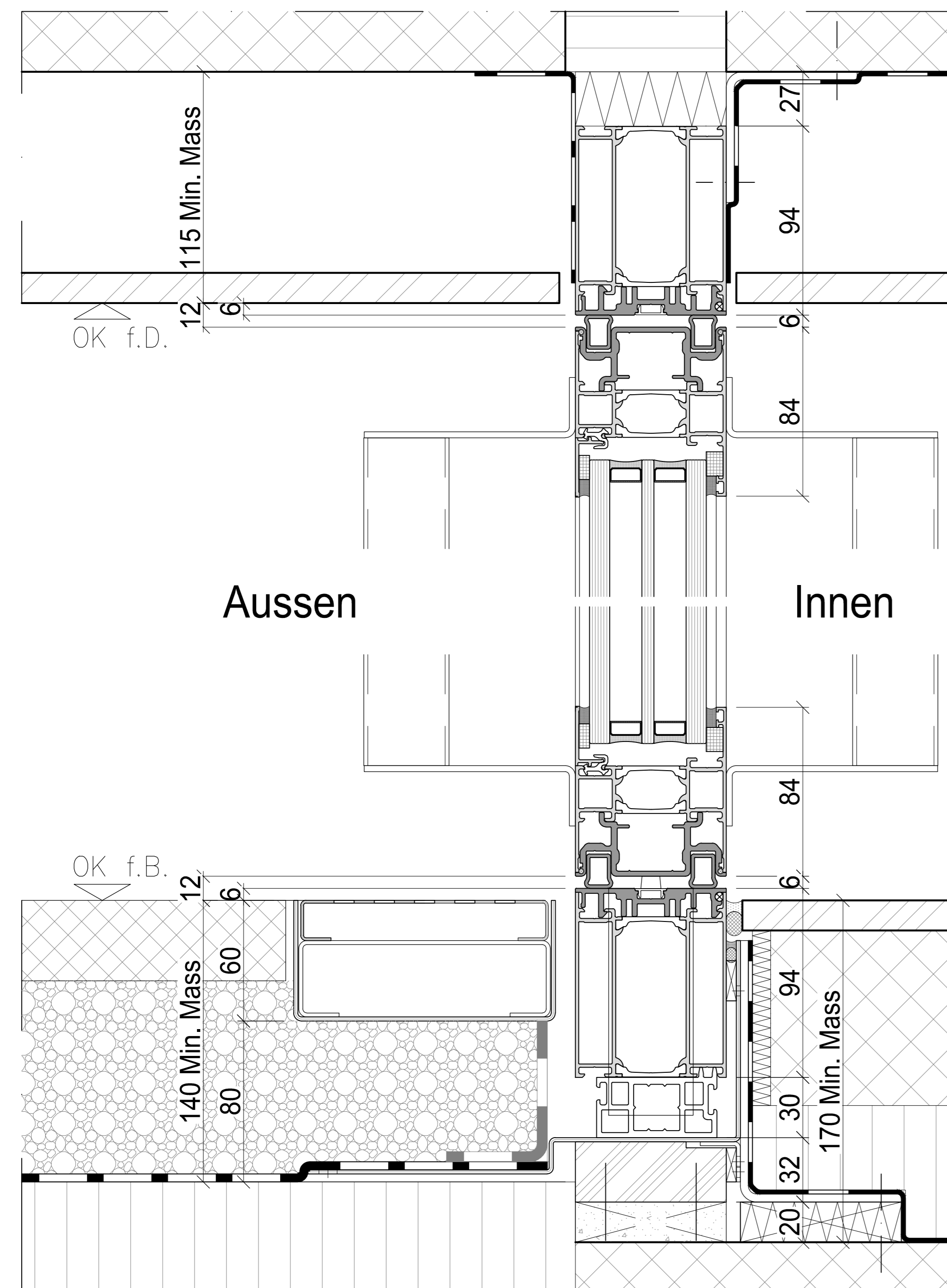
Schnitt B-B
