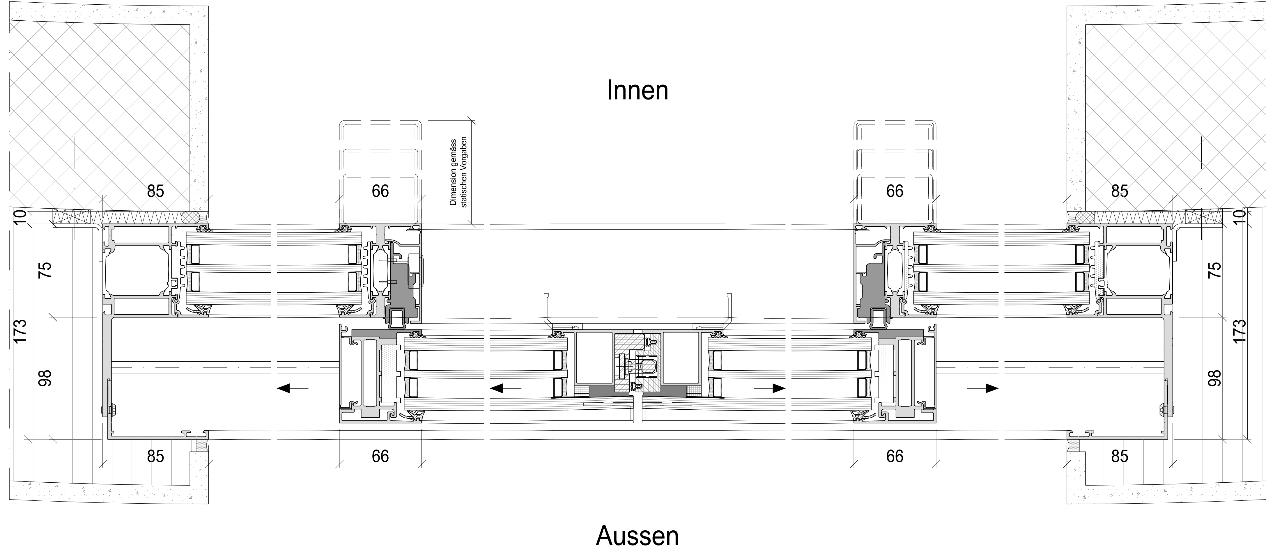
Schnitt C-C
