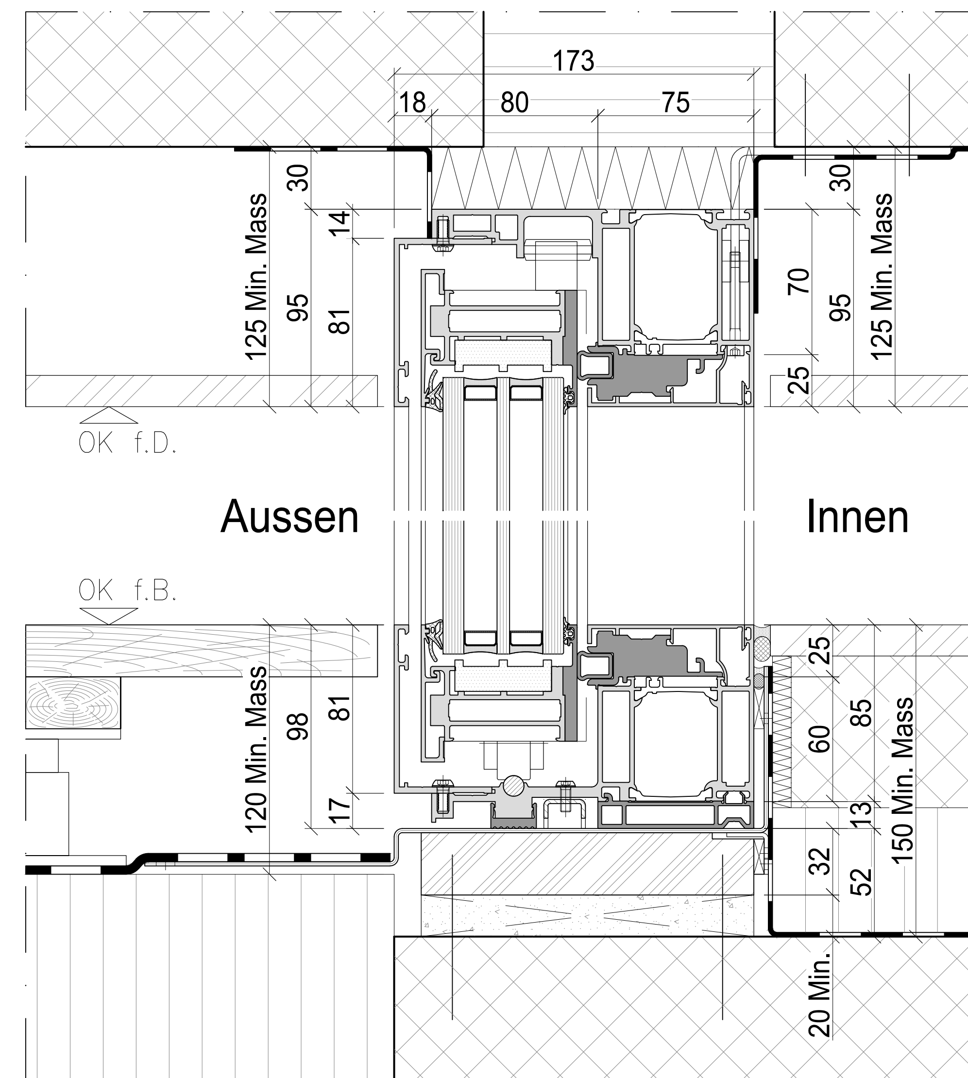
Schnitt B-B
