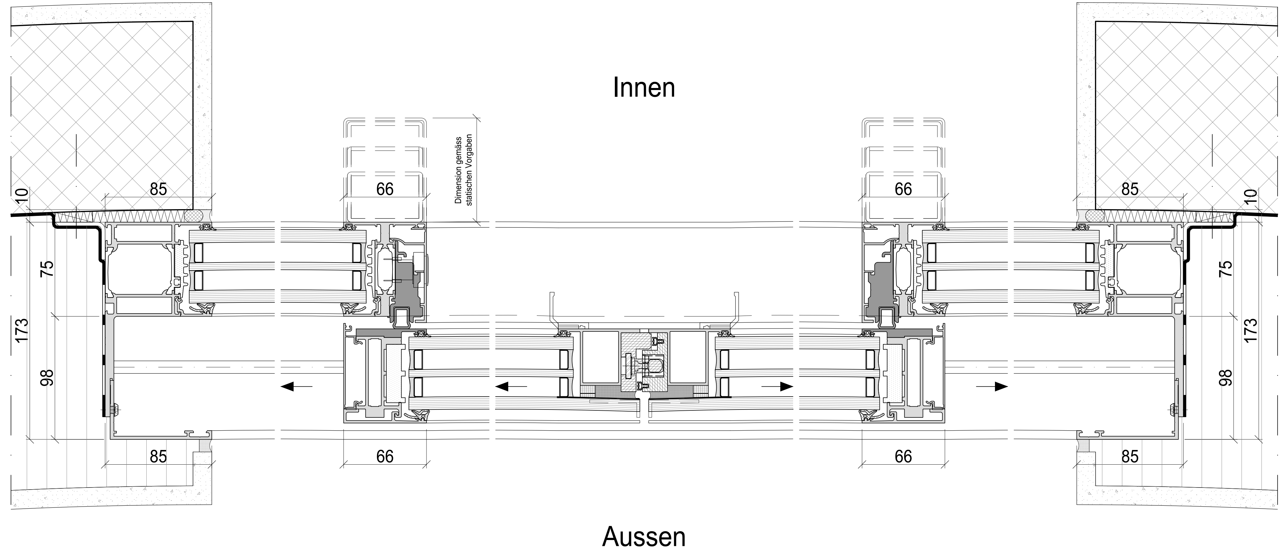
Schnitt C-C
