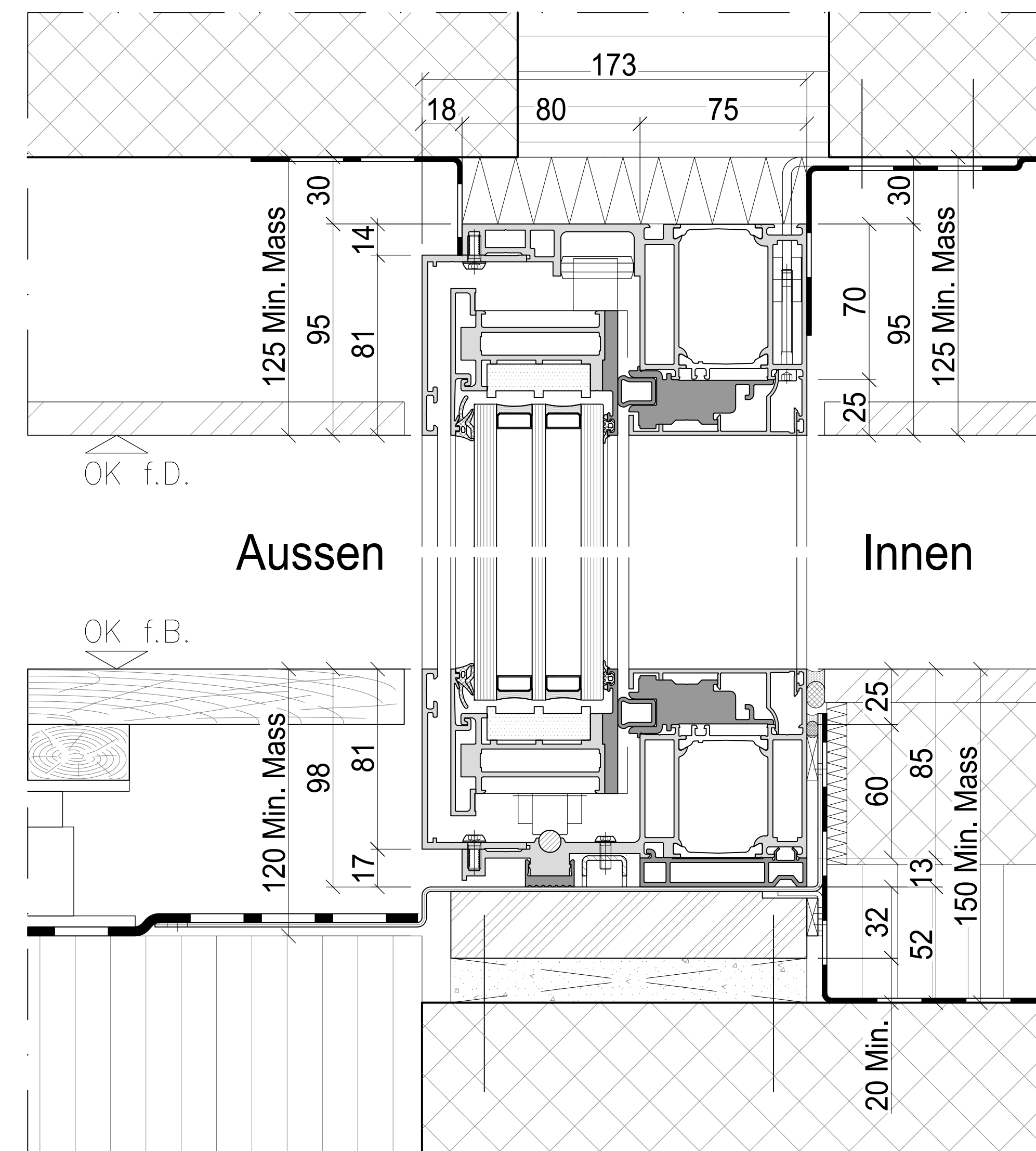
Schnitt B-B
