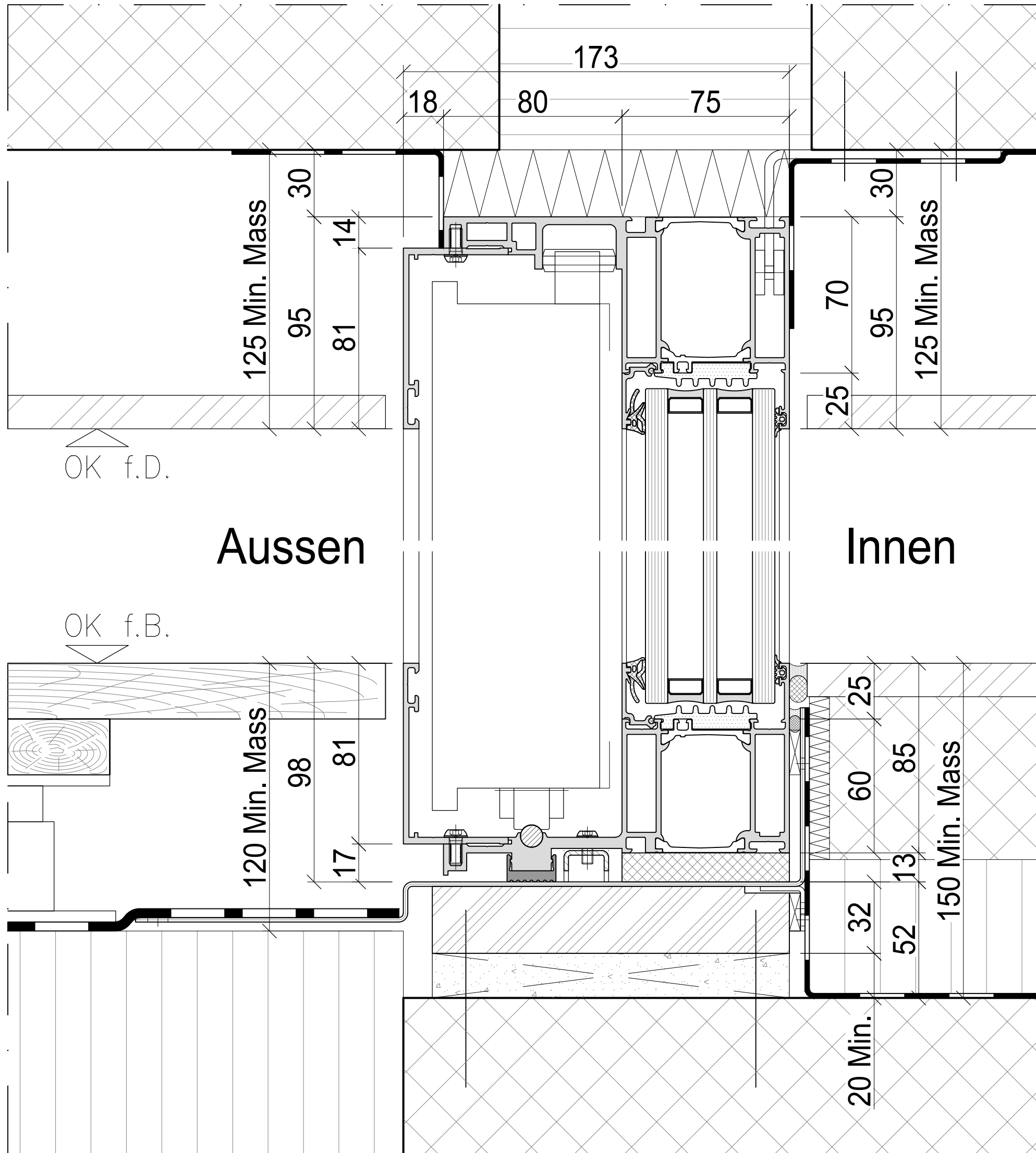
Schnitt A-A
