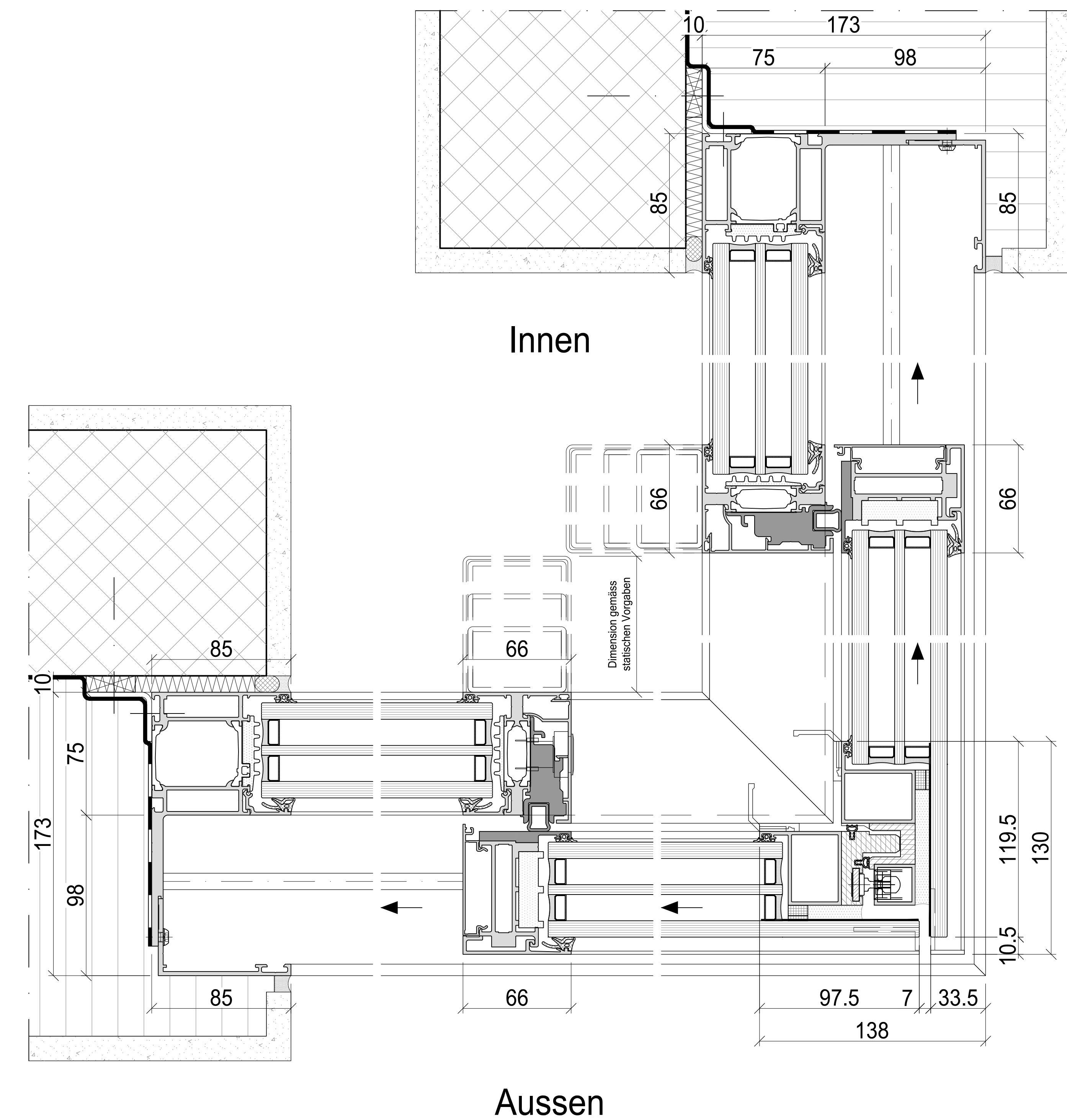
Schnitt C-C
