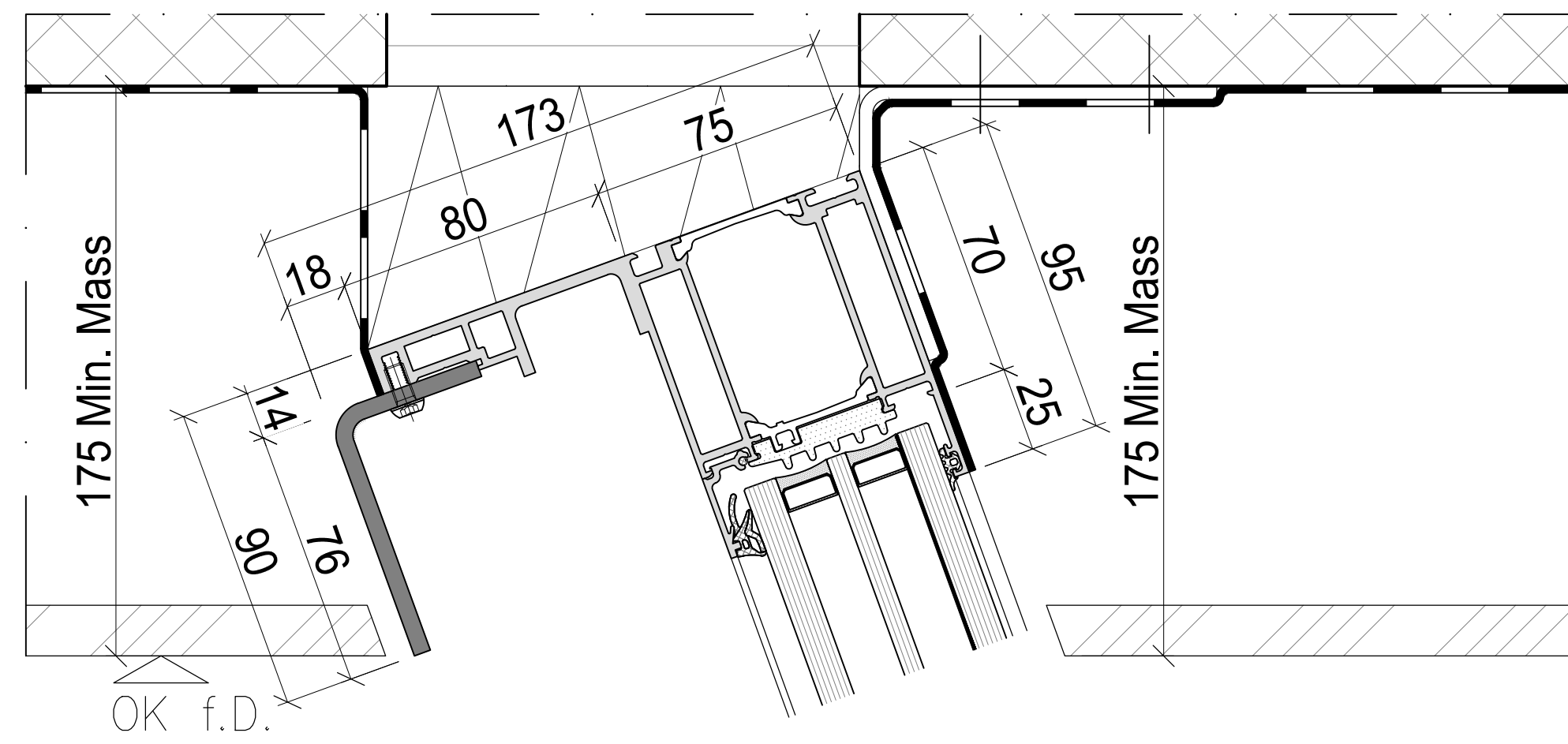
Schnitt A-A
