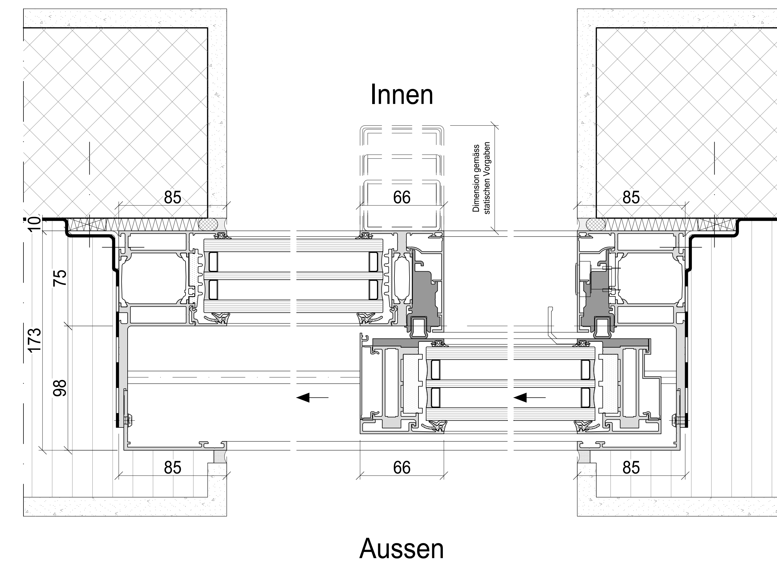
Schnitt C-C
