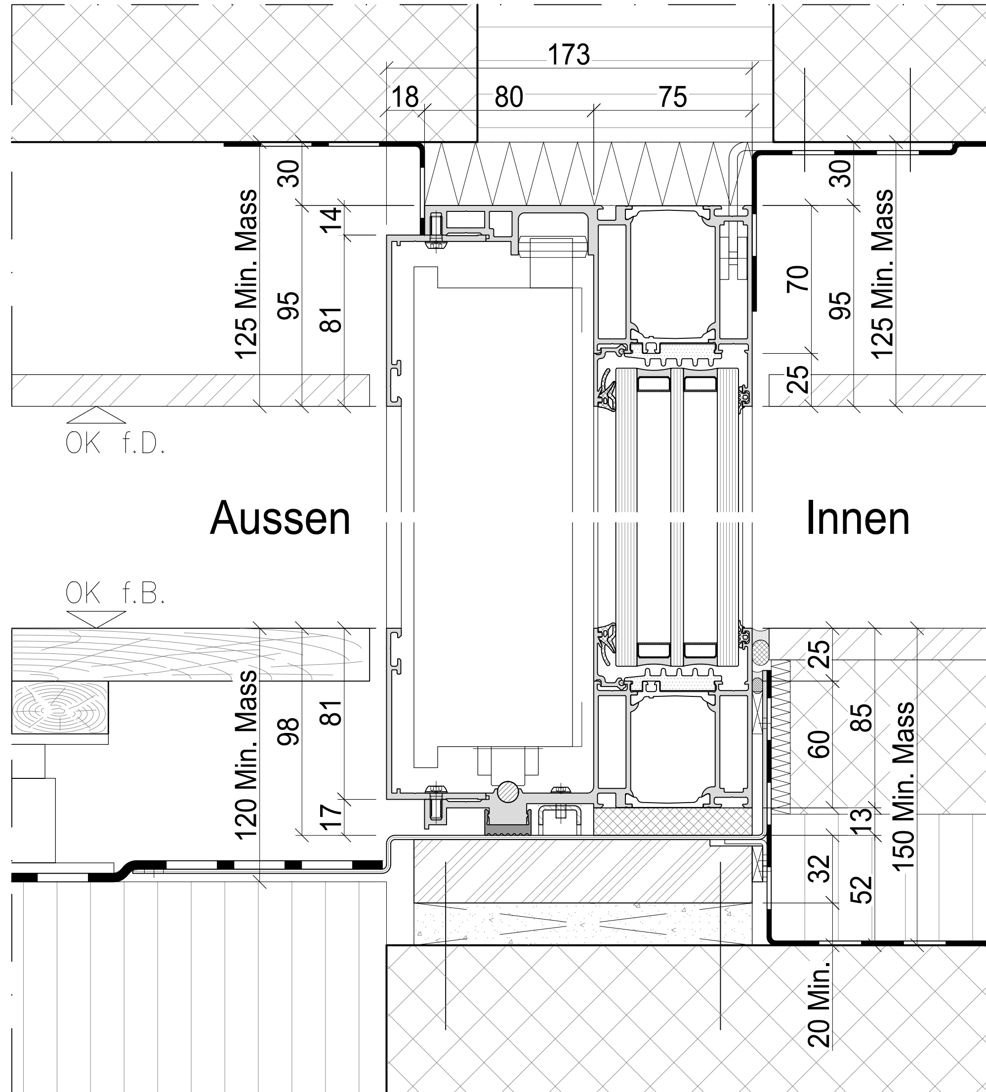
Schnitt A-A
