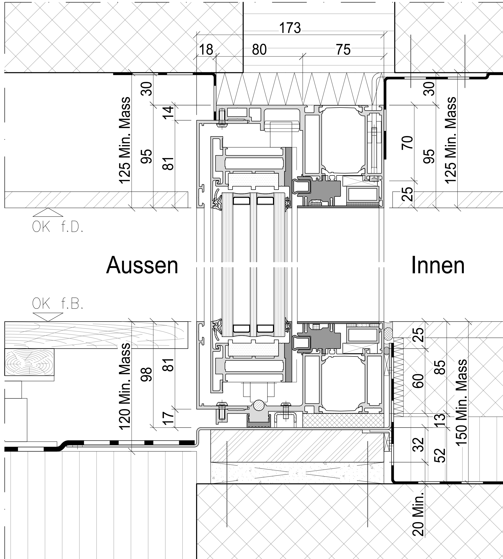
Schnitt B-E
