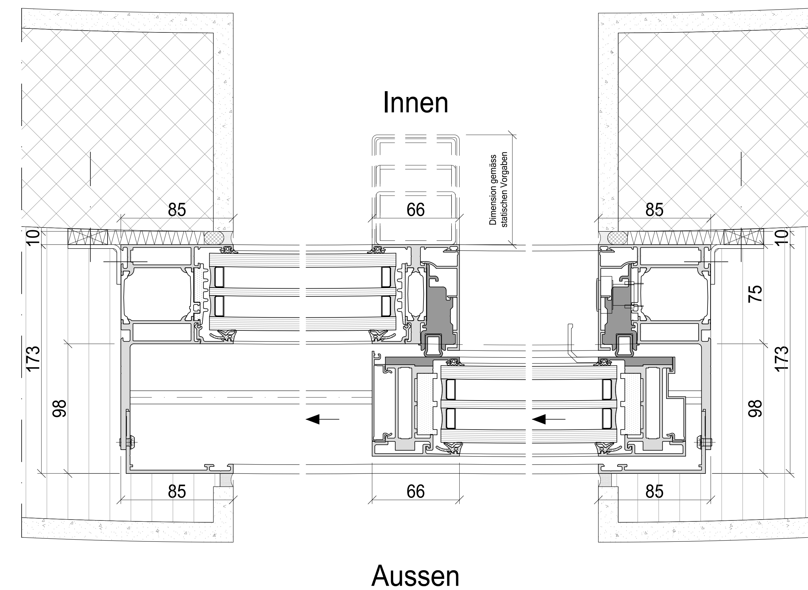
Schnitt C-C
