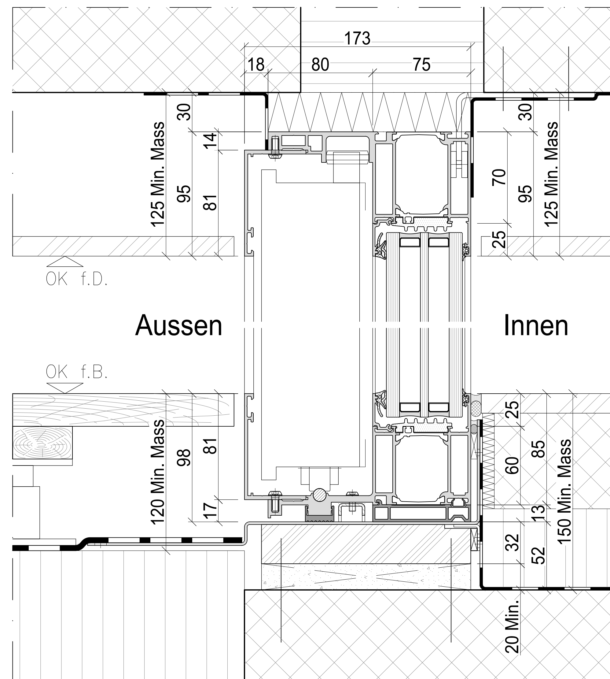
Schnitt A-A
