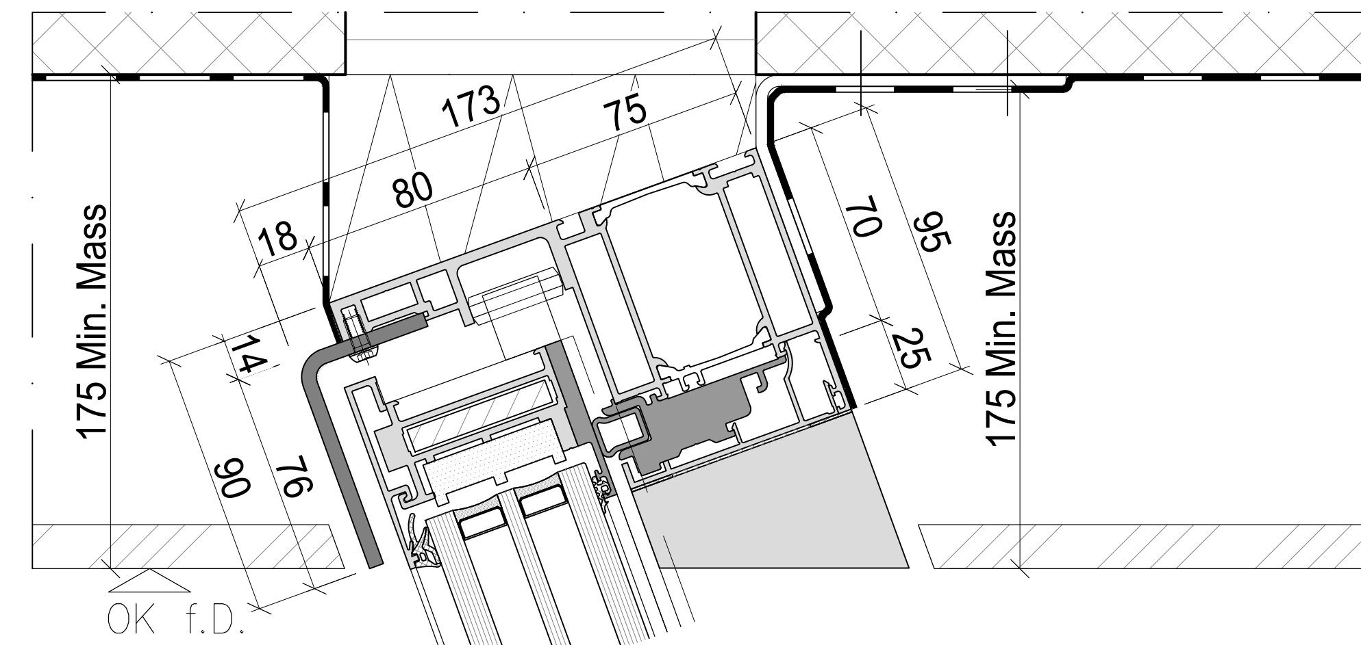
Schnitt B-B
