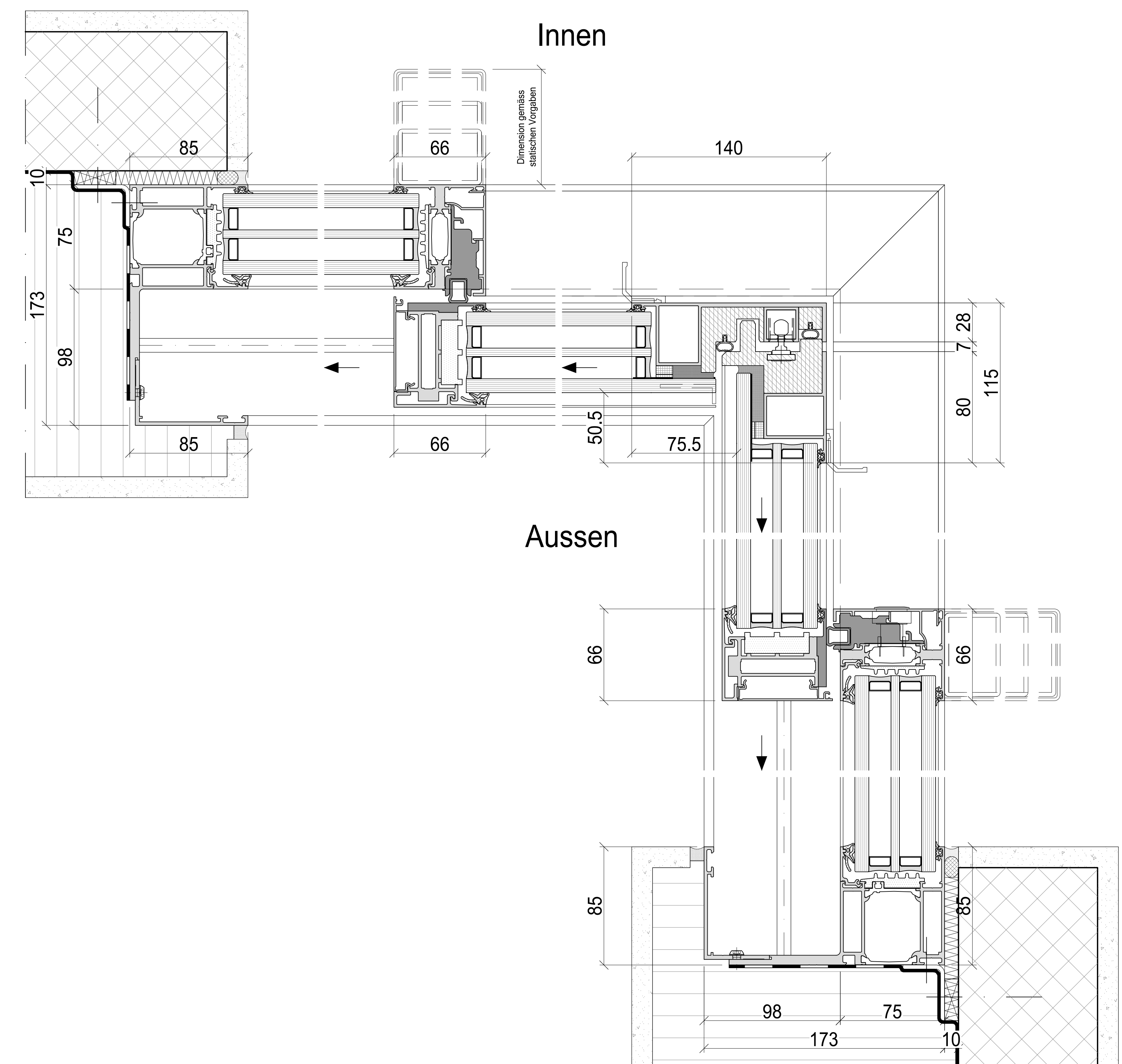
Schnitt C-C
