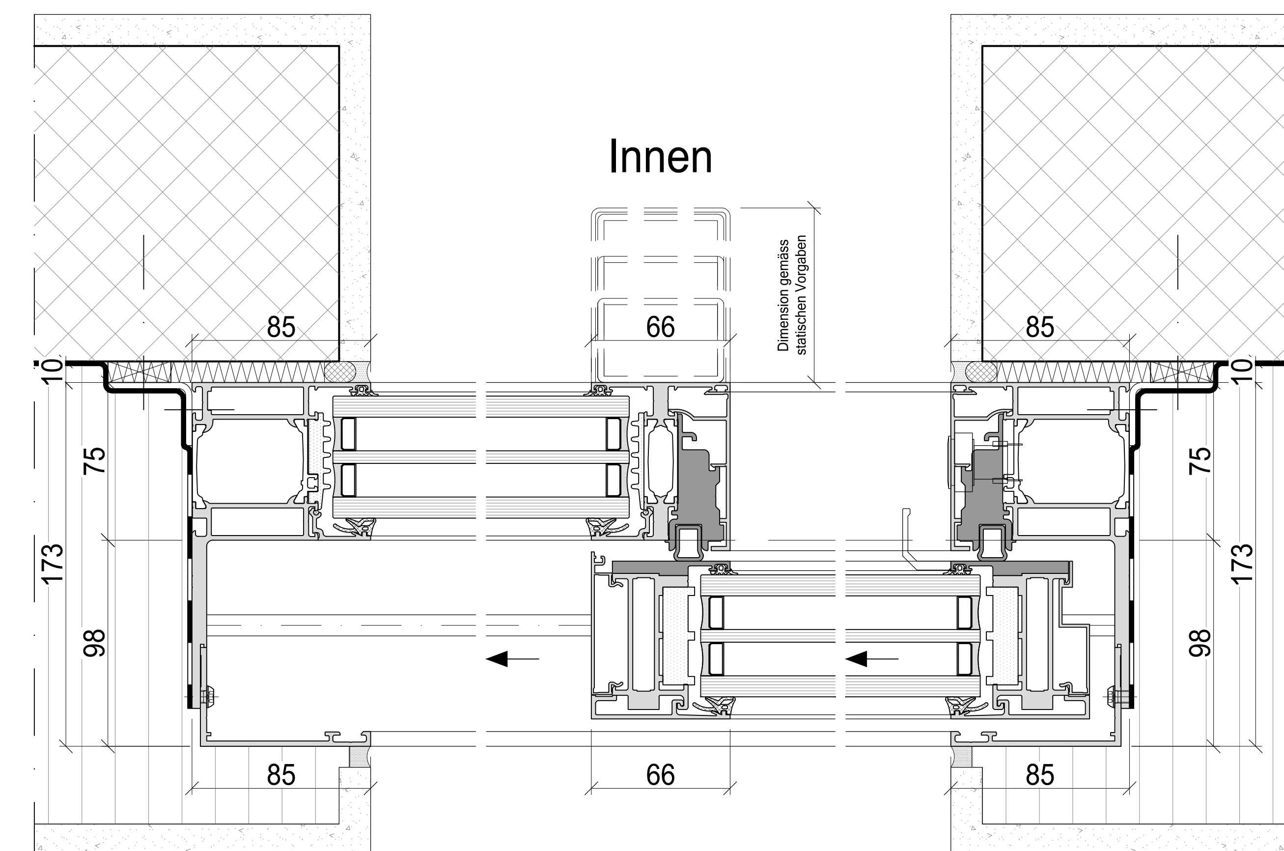
Schnitt C-C
