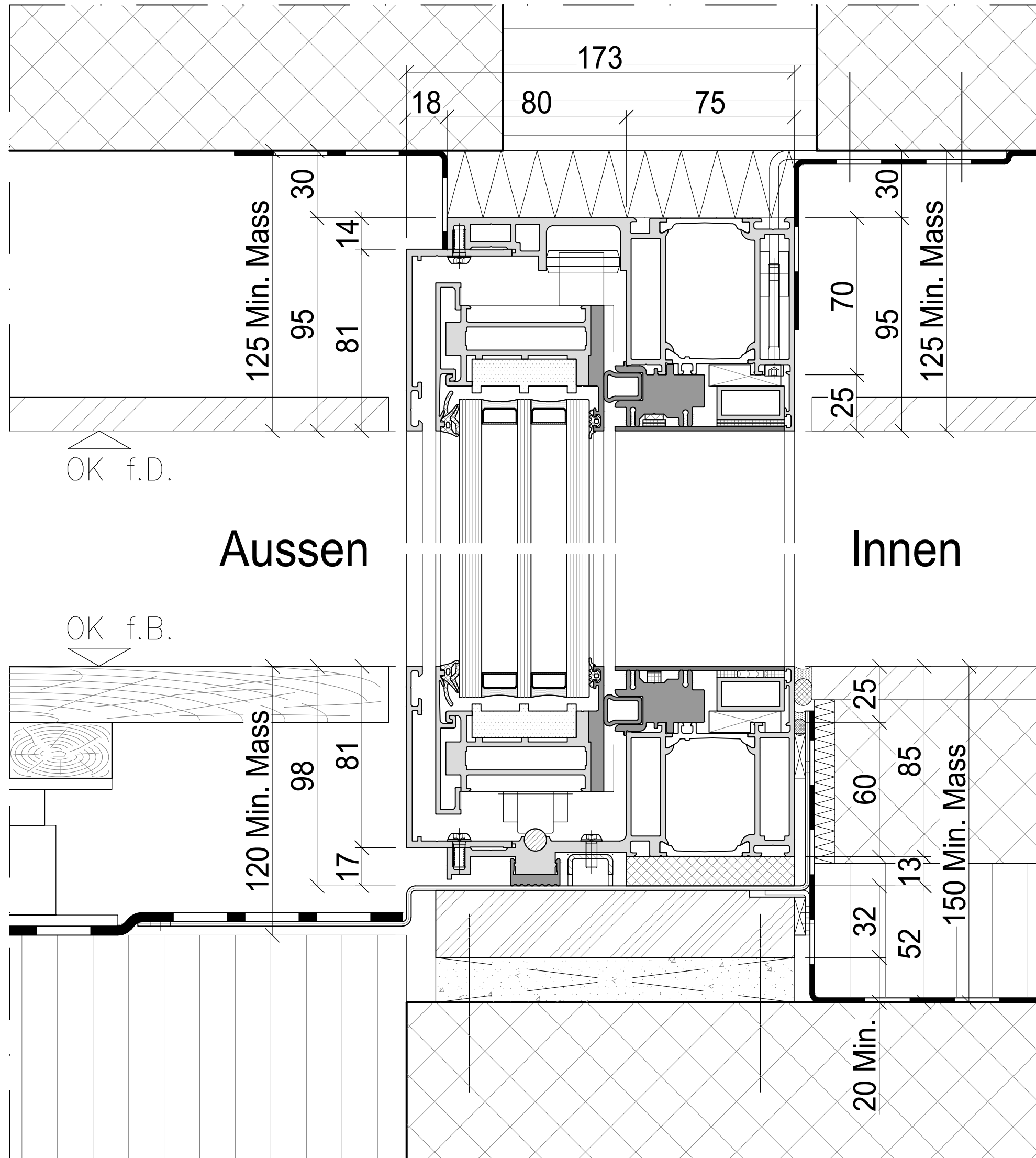
Schnitt B-B
