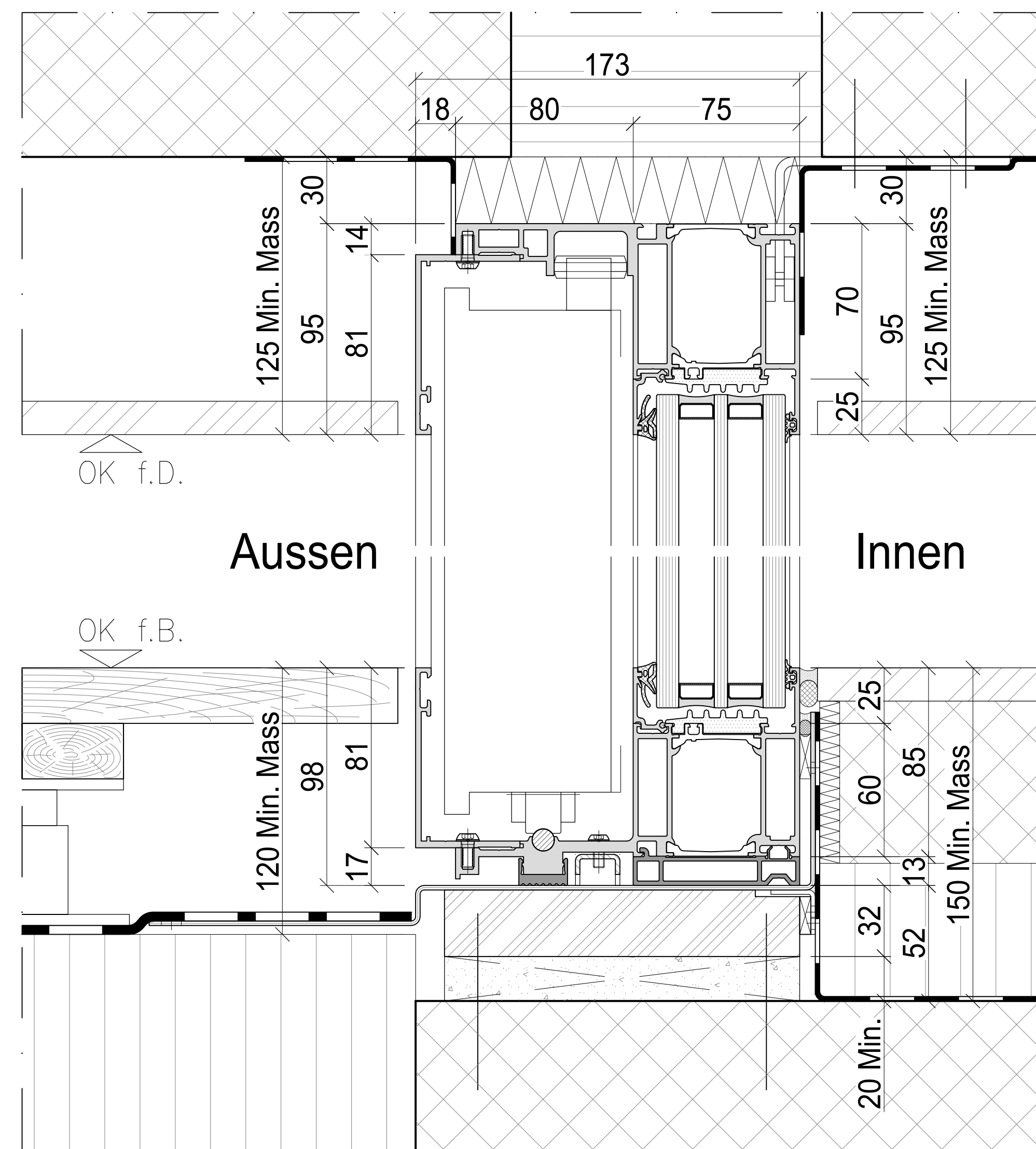
Schnitt A-A
