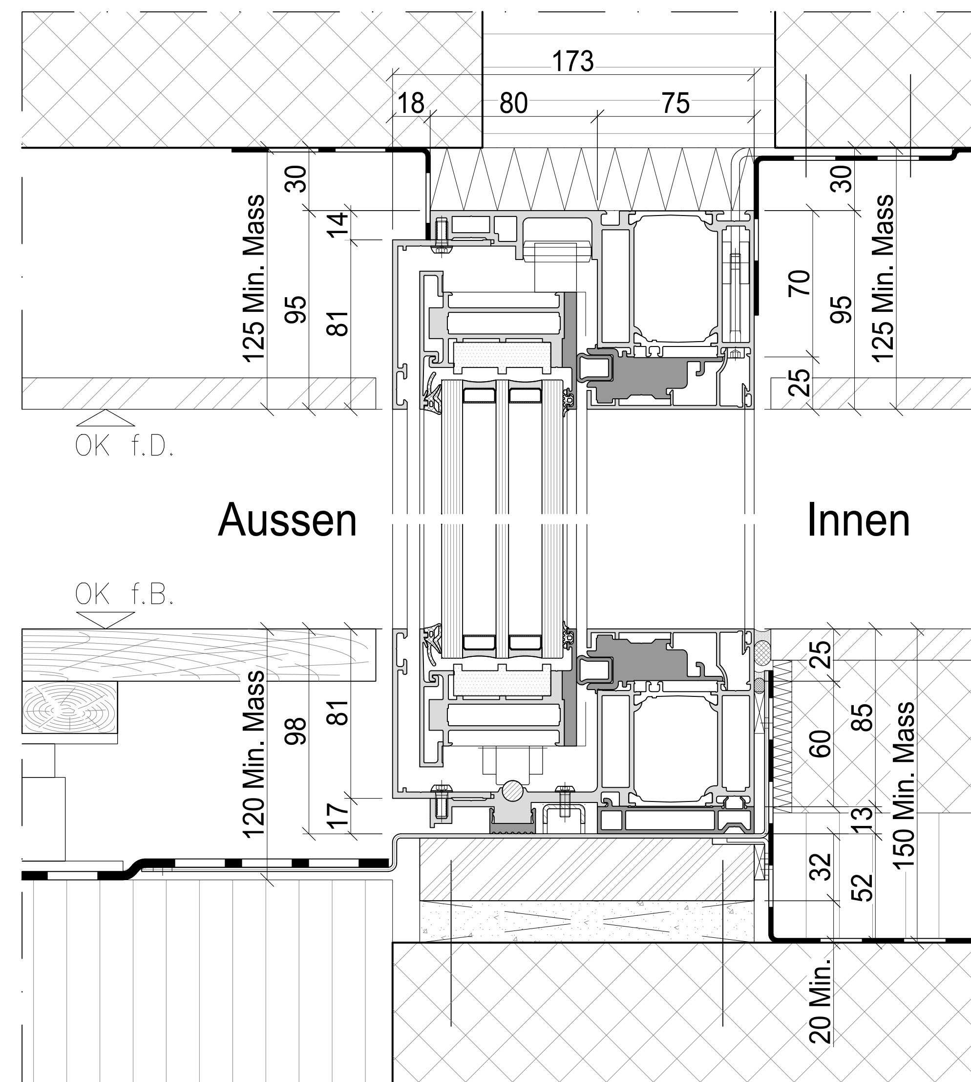
Schnitt B-B
