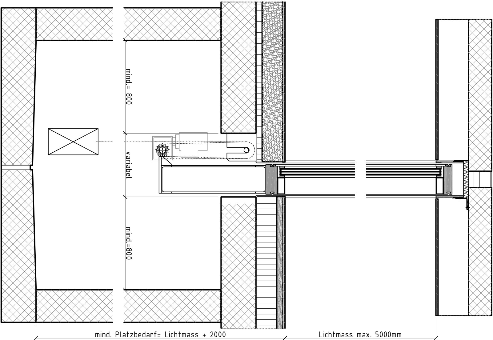
Schnitt A-A
