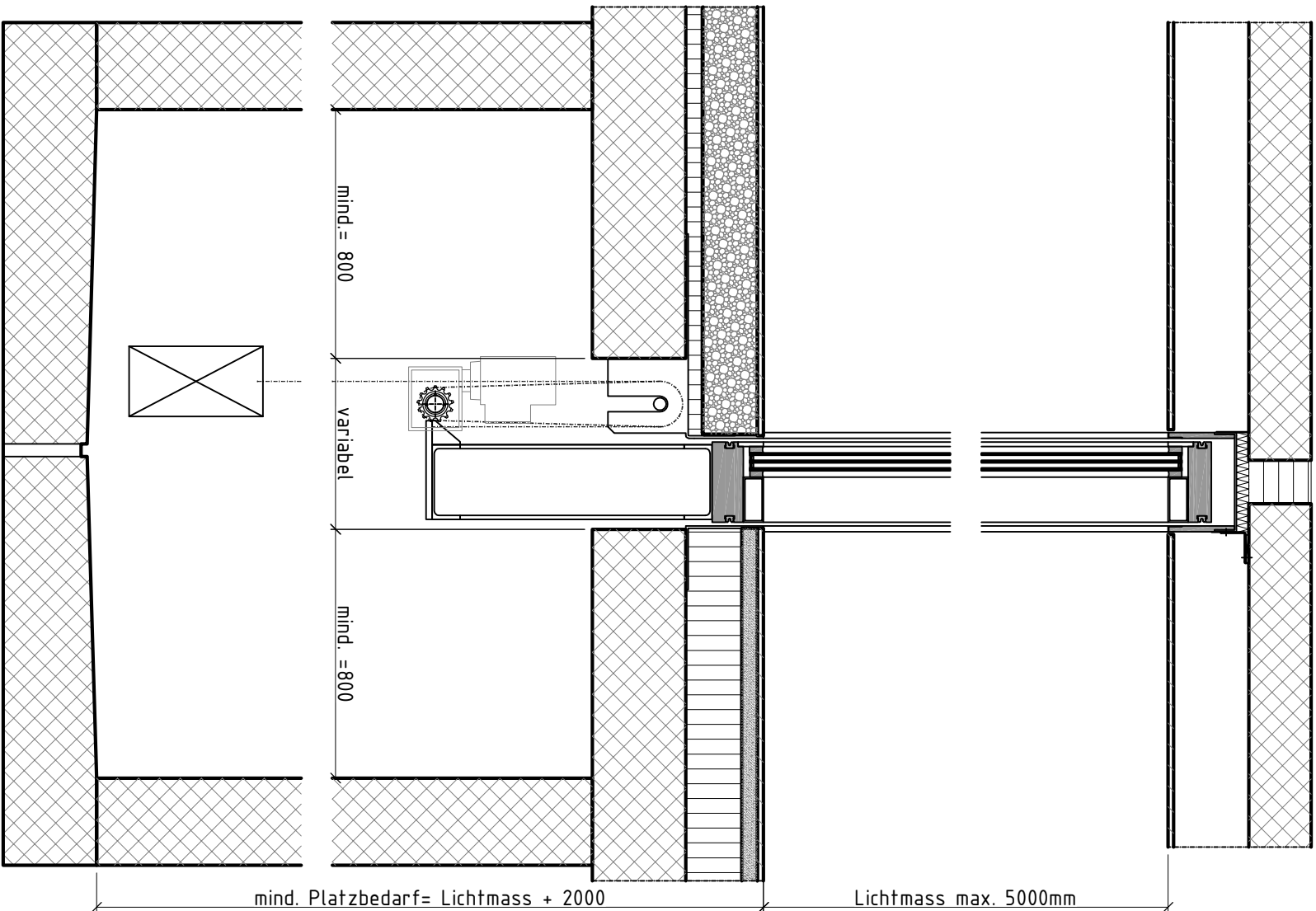
Schnitt A-A
