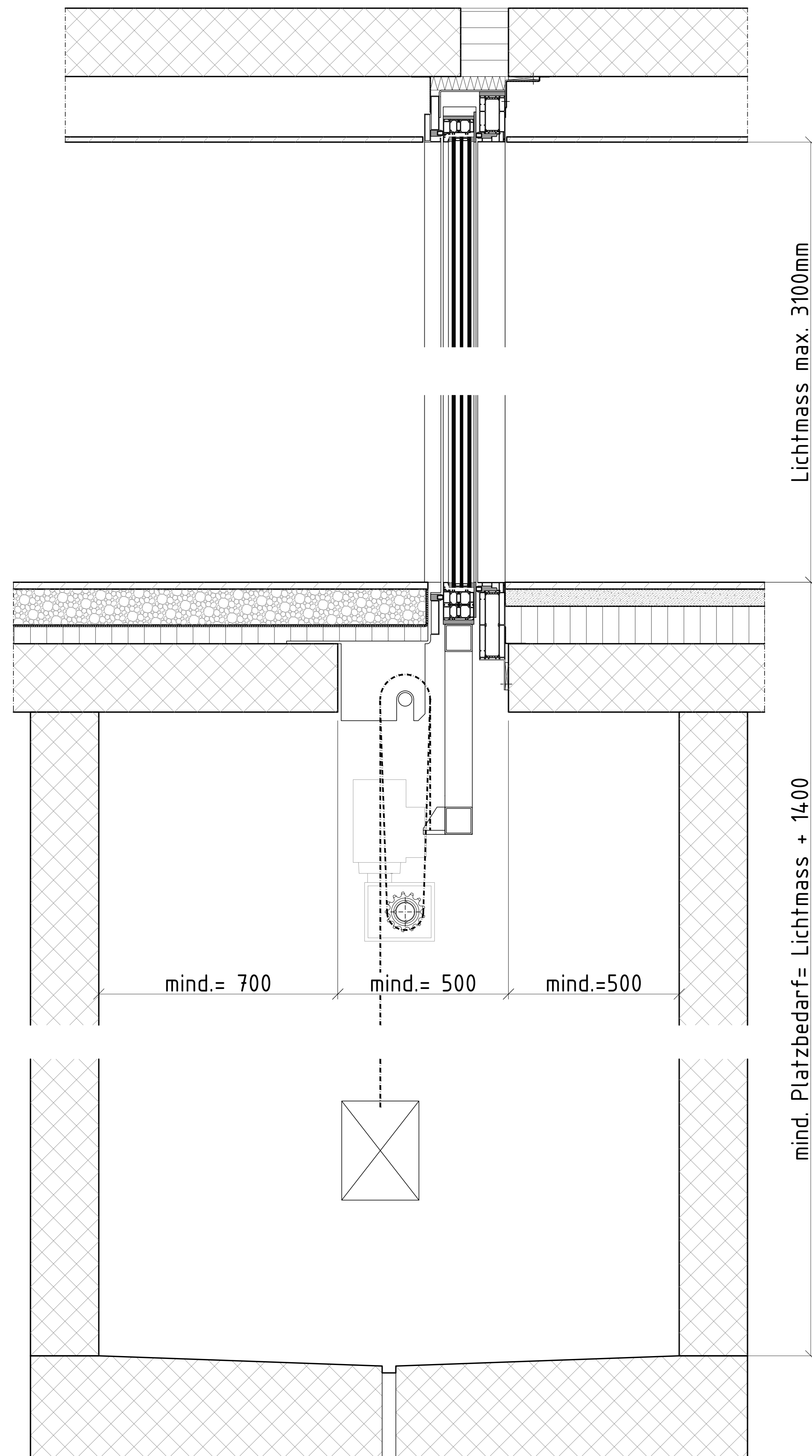
Schnitt A-A
