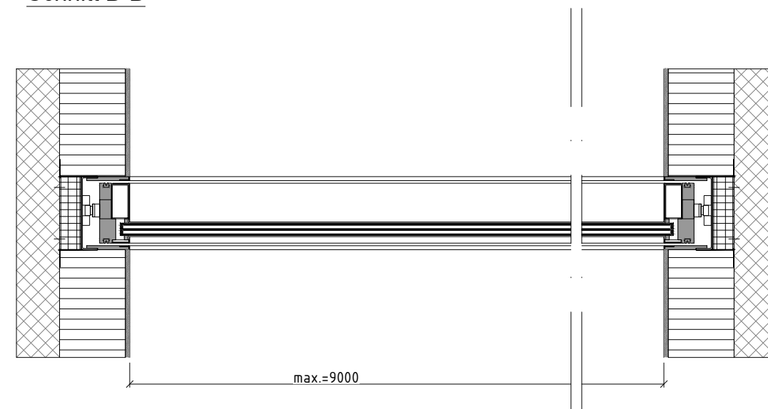
Schnitt B-B
