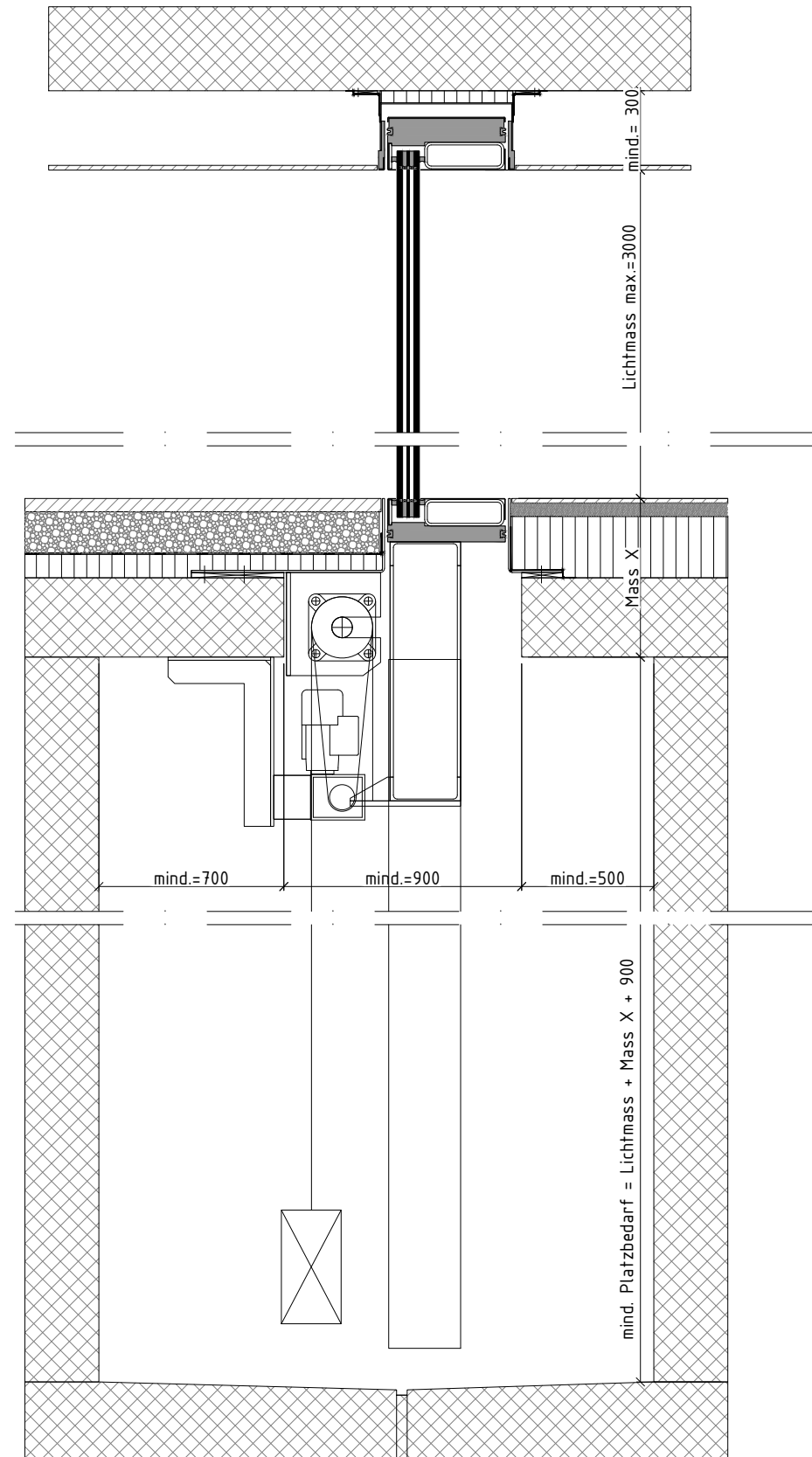
Schnitt A-A
