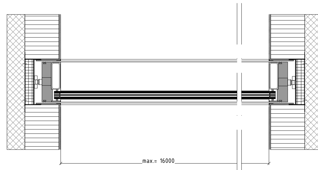
Schnitt B-B
