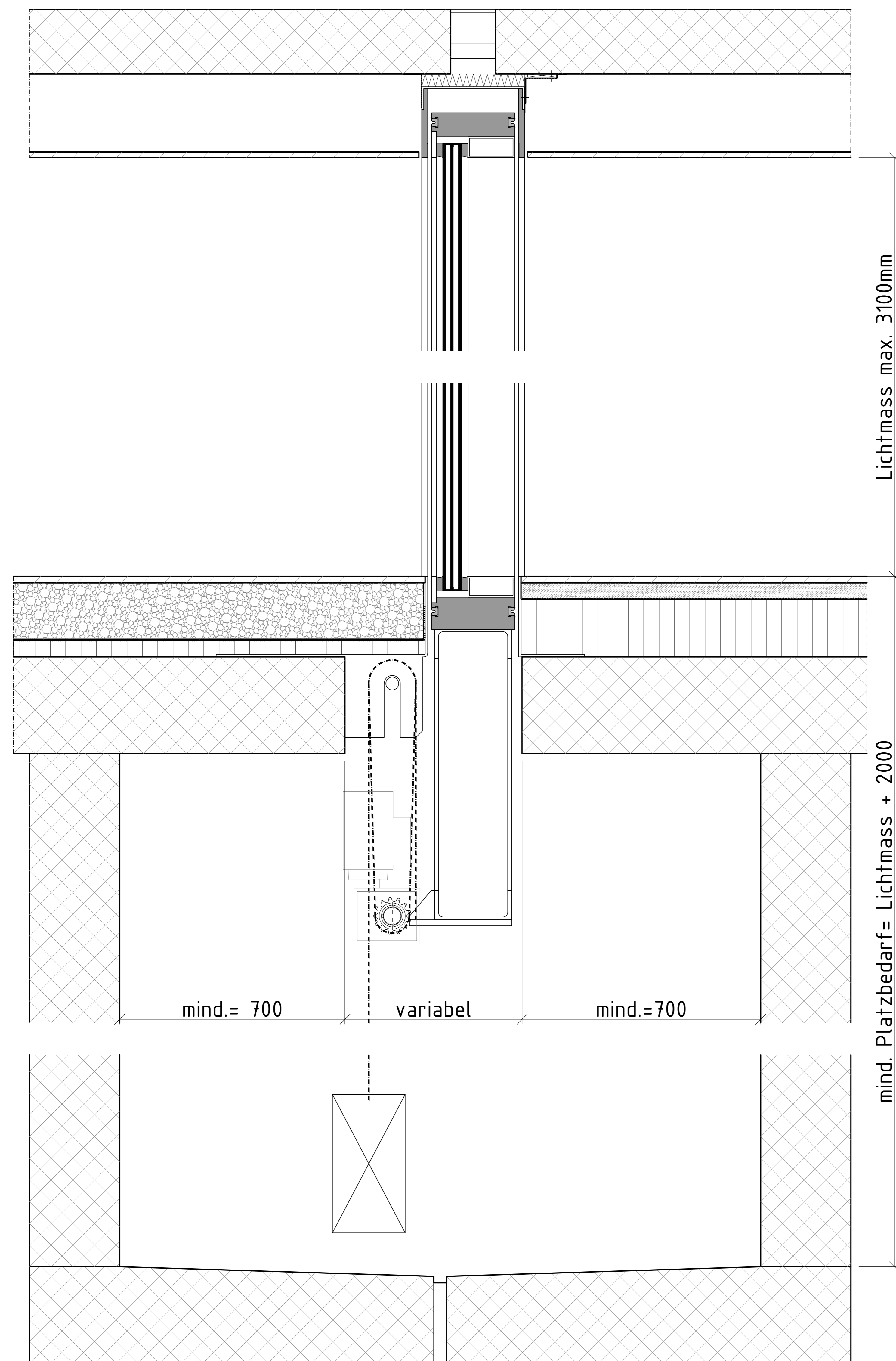
Schnitt A-A
