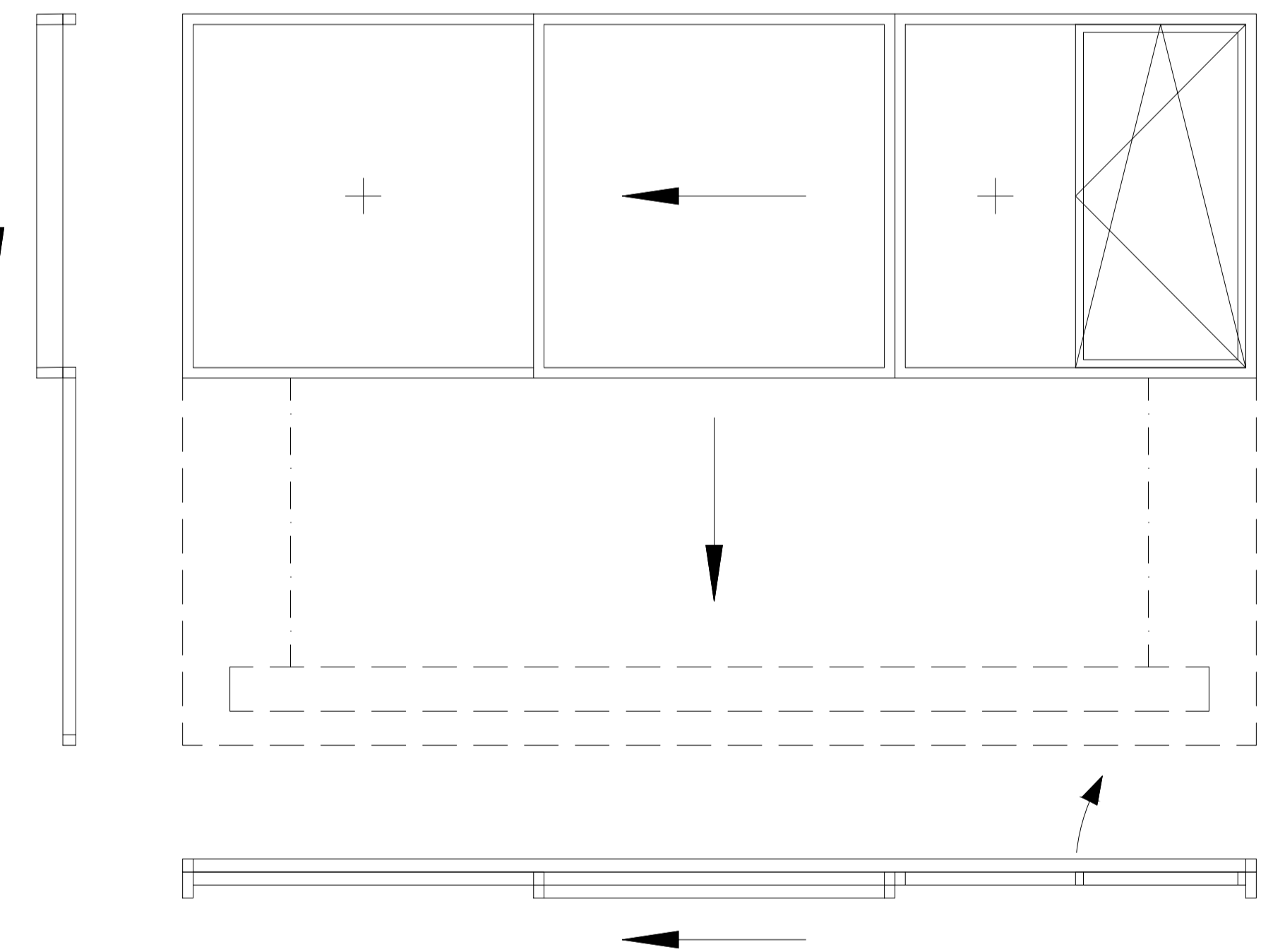
Senkfenster Schiebefenster Schema A und Drehkipp-Fenster
