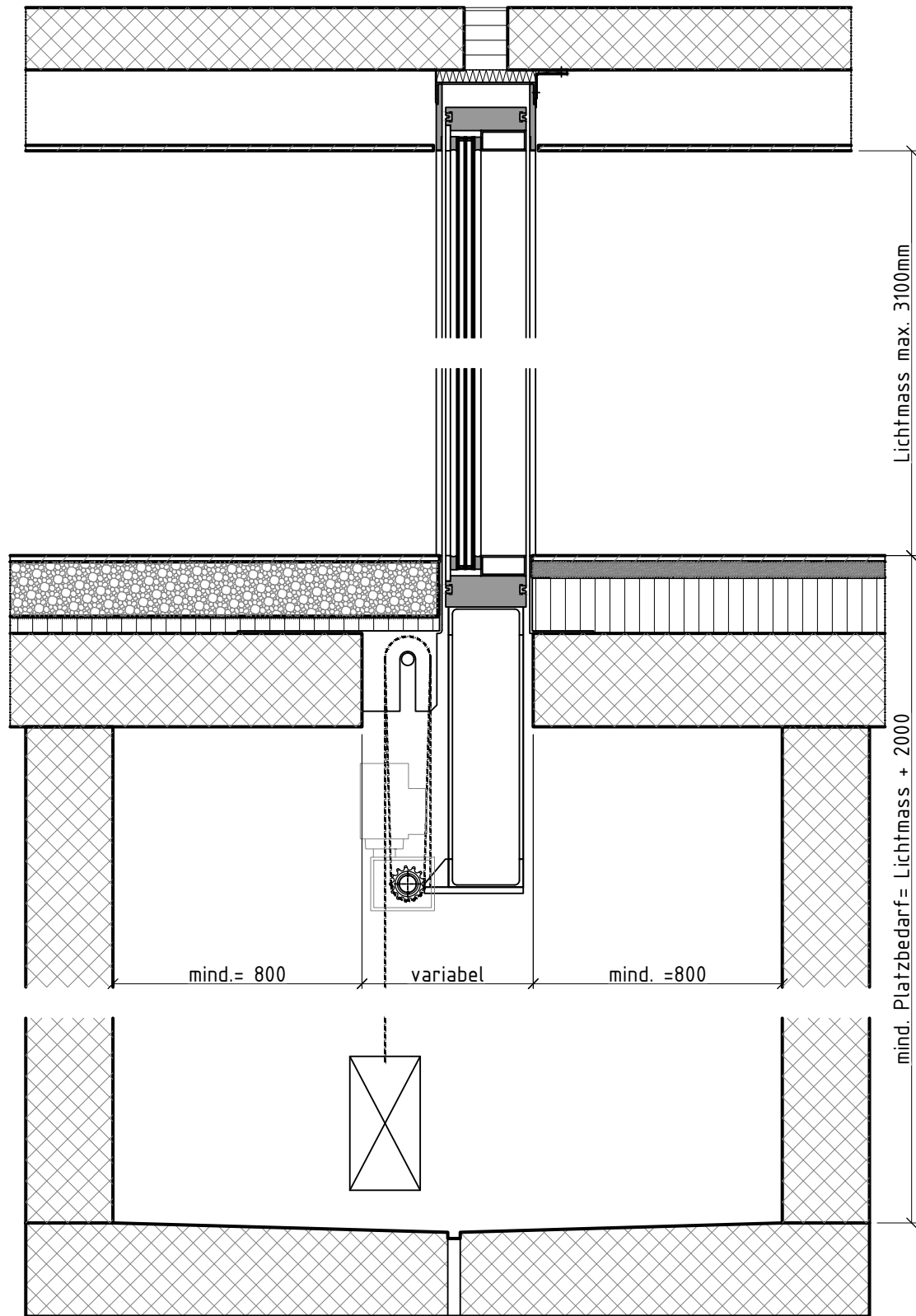
Schnitt A-A
