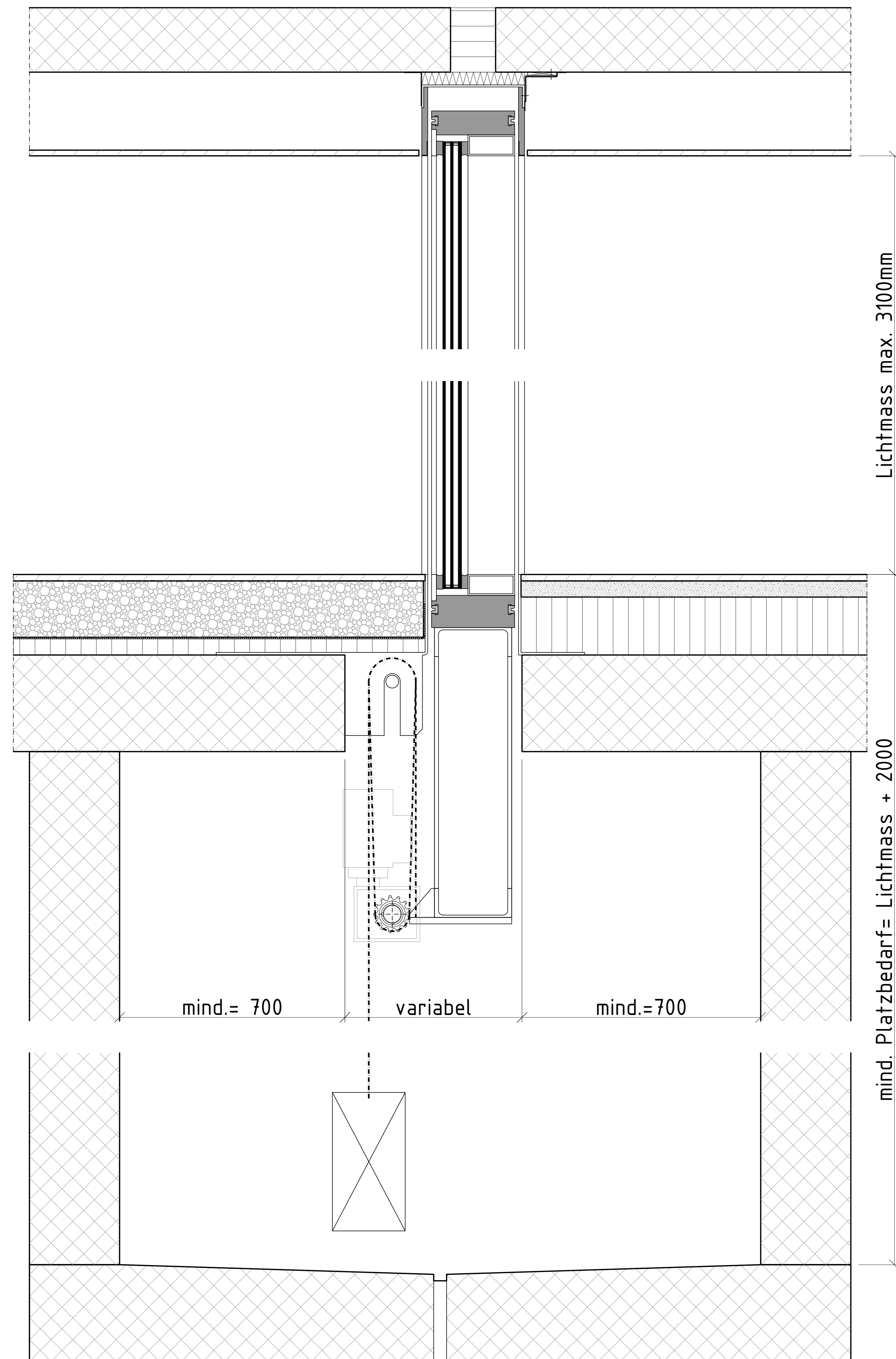
Schnitt A-A
