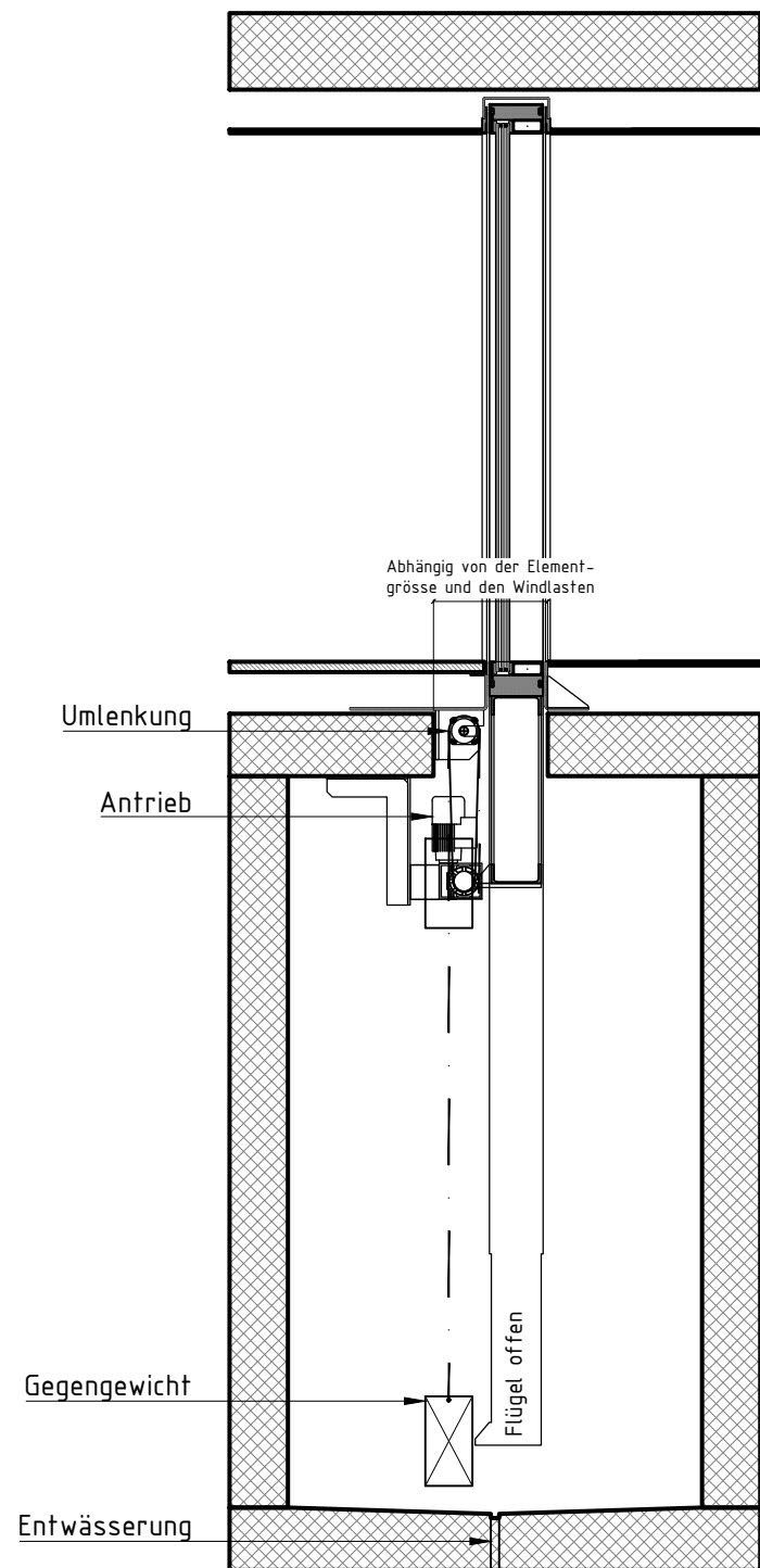
Vertikalschnitt
